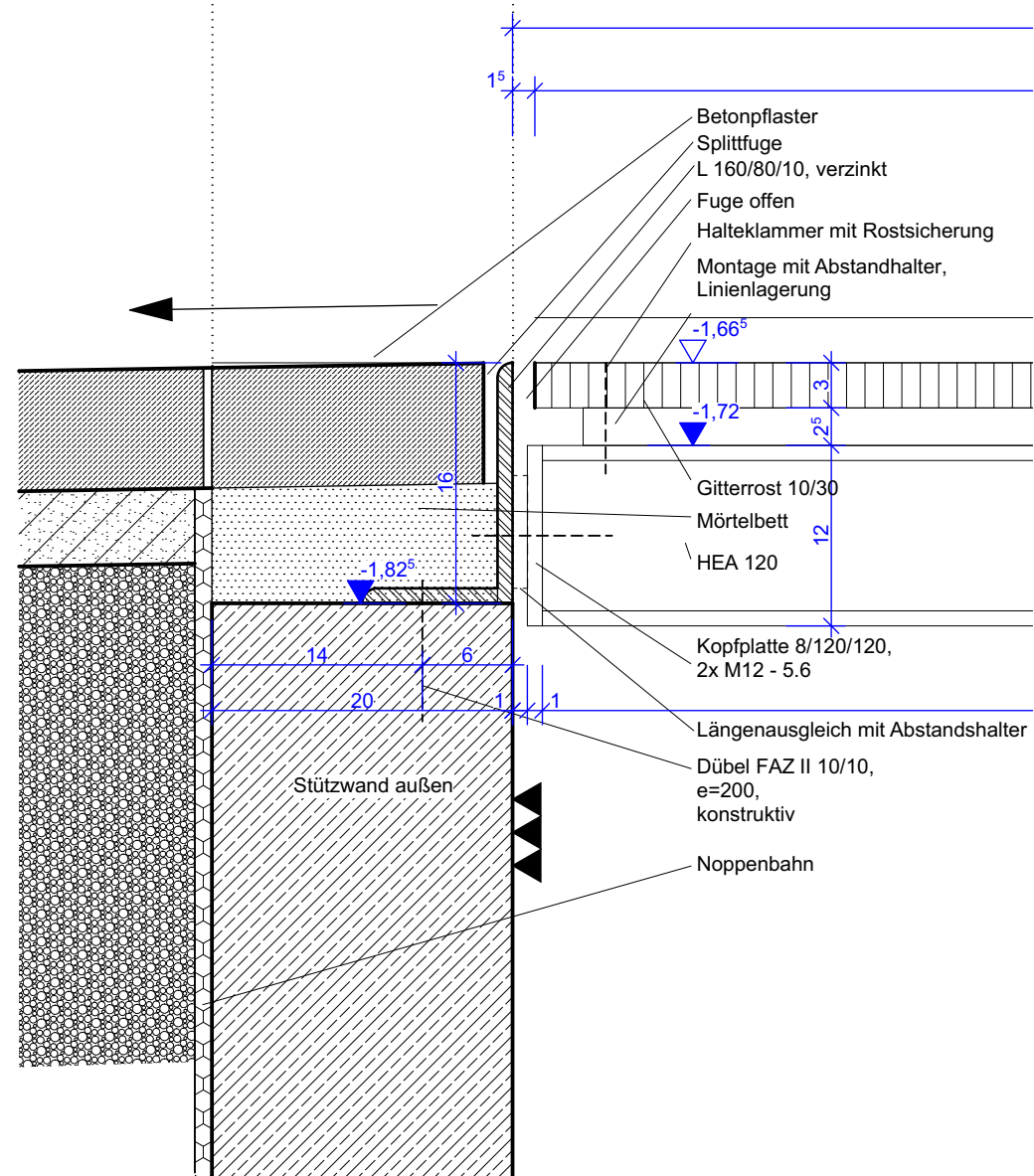
Vertikalschnitt Stützwand außen - Bereich Gitterrostzugang
