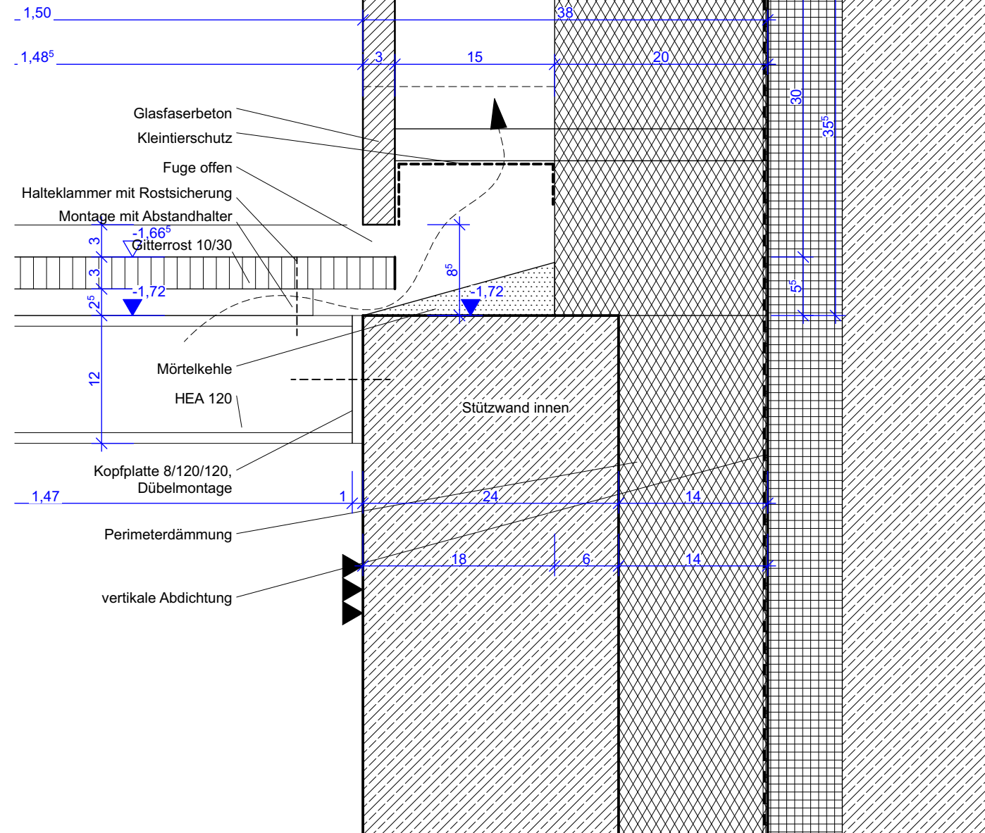
Vertikalschnitt Stützwand innen
