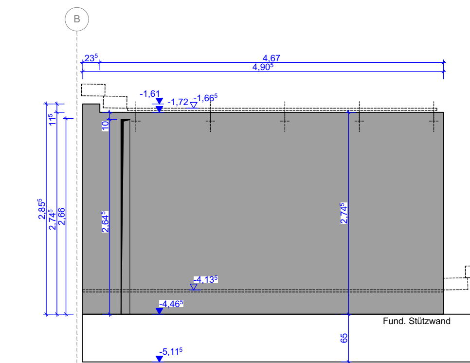
Stützwall innen Ansicht M. 1/50
