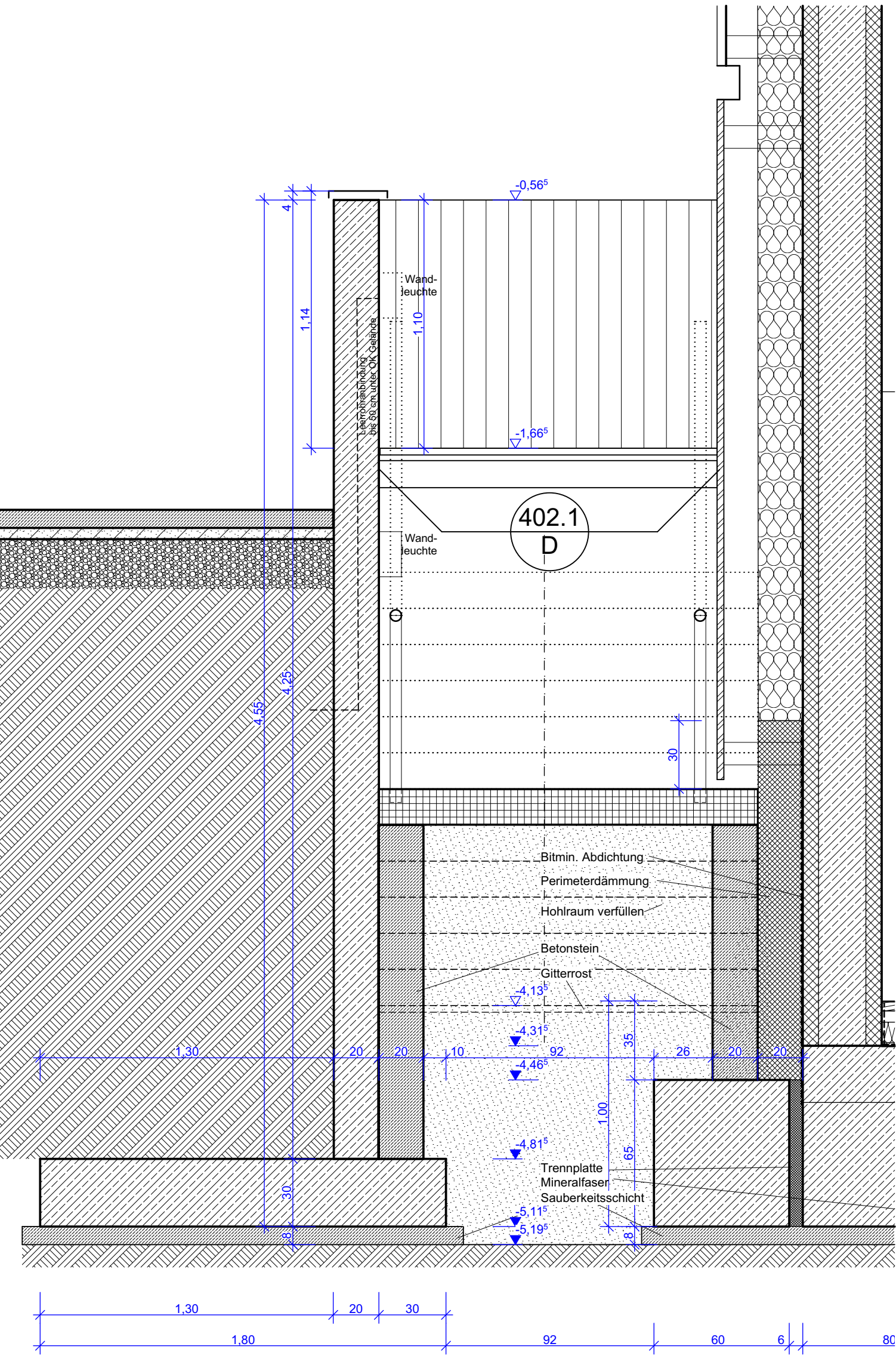
Vertikalschnitt b-b
