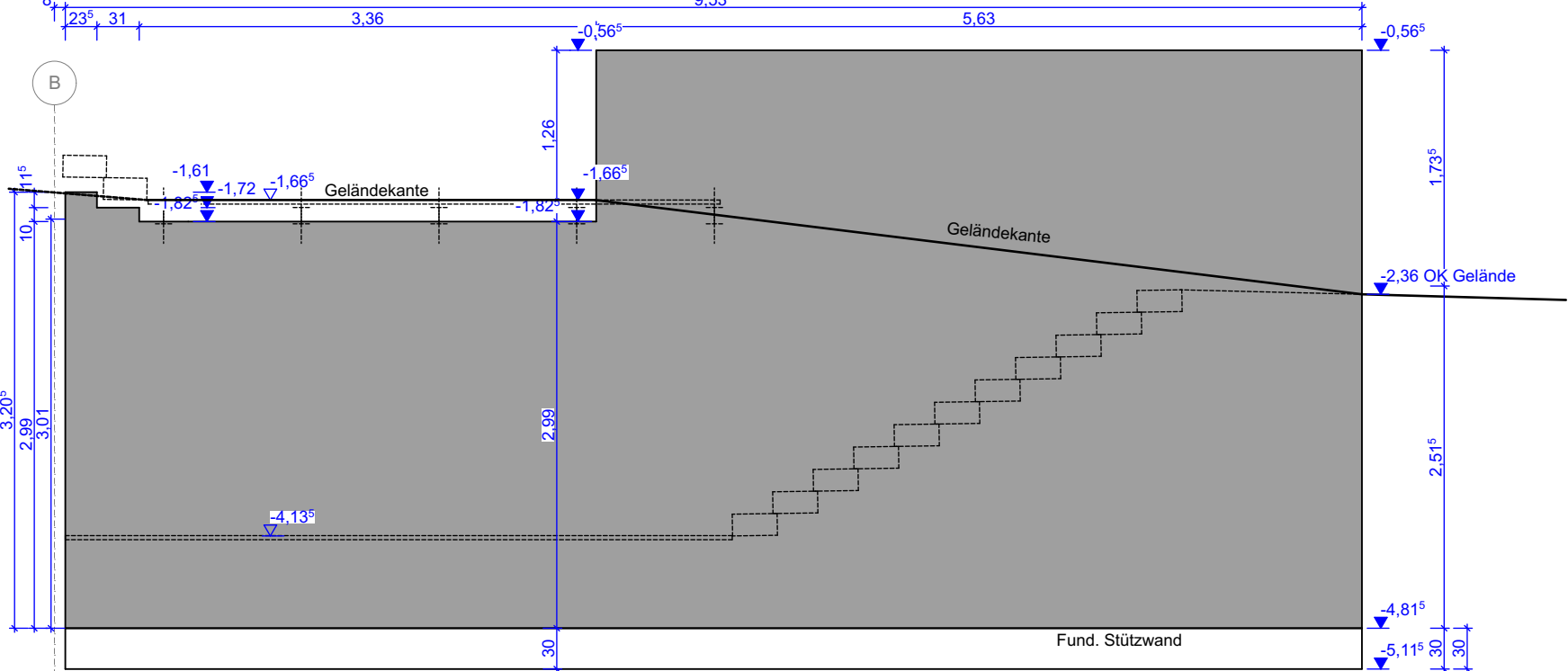
Stützwall außen Ansicht M. 1/50
