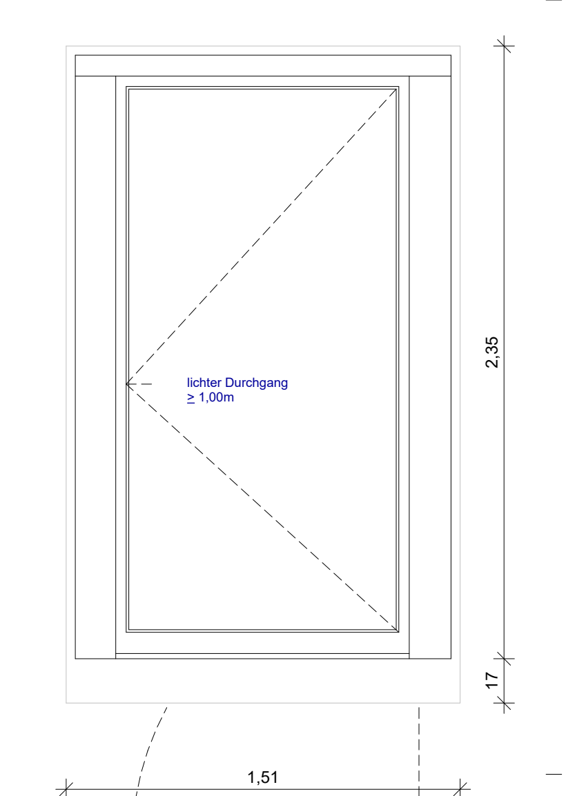
POS. 1.2.60 MEI-6 Aluminium-Türelement o.A.
