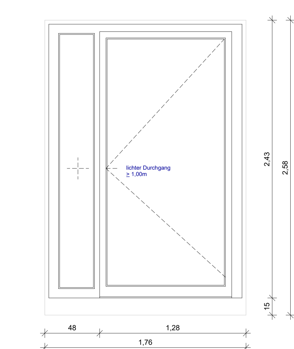
POS. 1.2.50 MEI-5 Aluminium-Türelement o.A.
