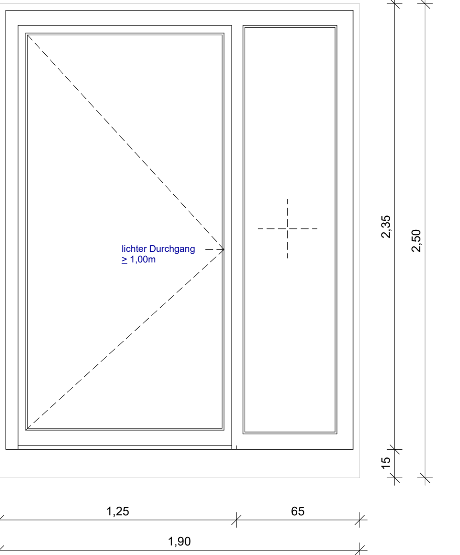
POS. 1.2.30 MEI-3 Aluminium-Türelement o.A.
