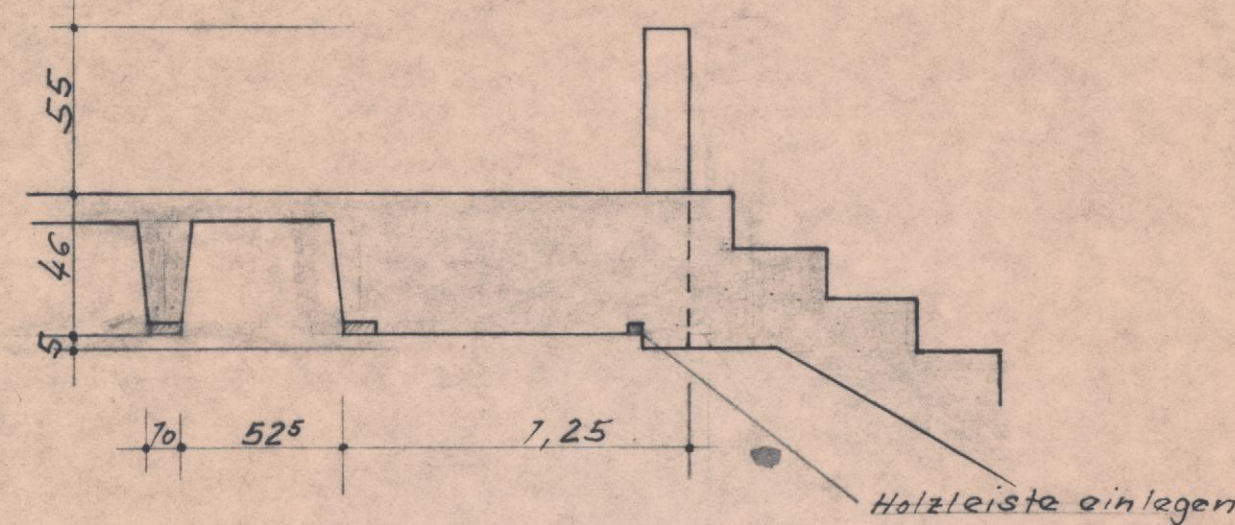
Schnitt b-b M. 1:25
