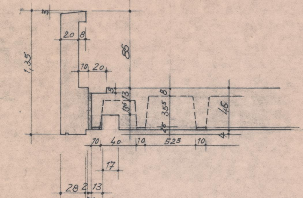
Schnitt c-c M. 1:25
