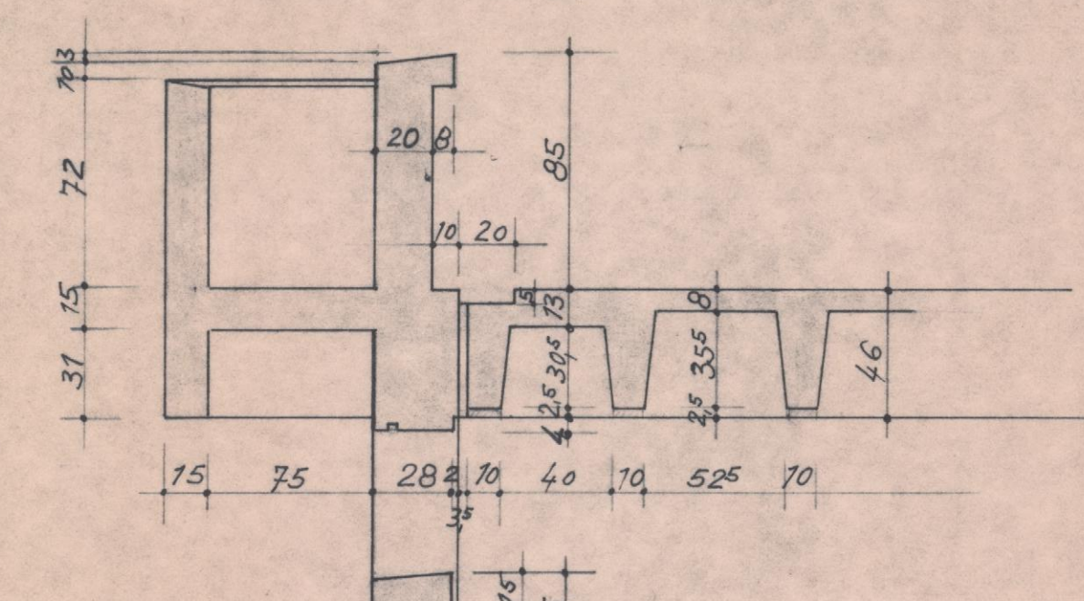
Schnitt g-g M. 1:25
