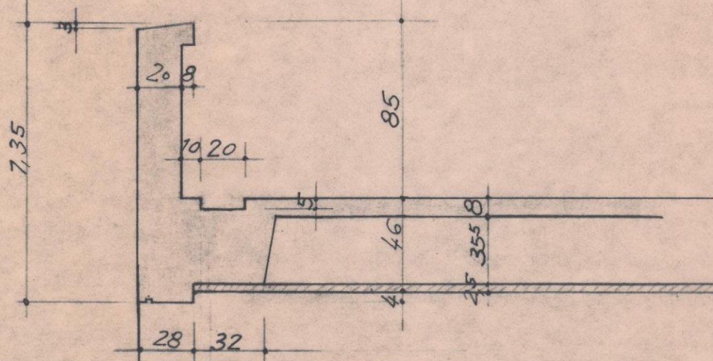
Schnitt durch Fensterband M. 1:25
