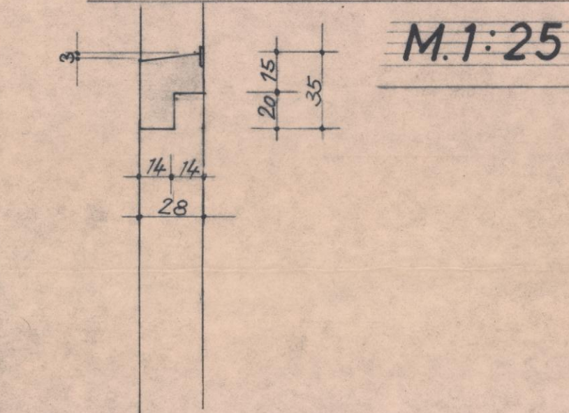
Schnitt c-c M. 1:25
