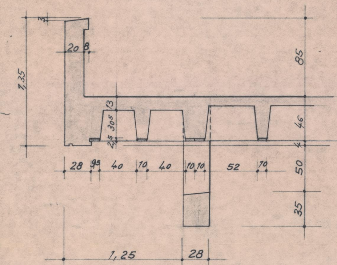
Schnitt d-d M. 1:25
