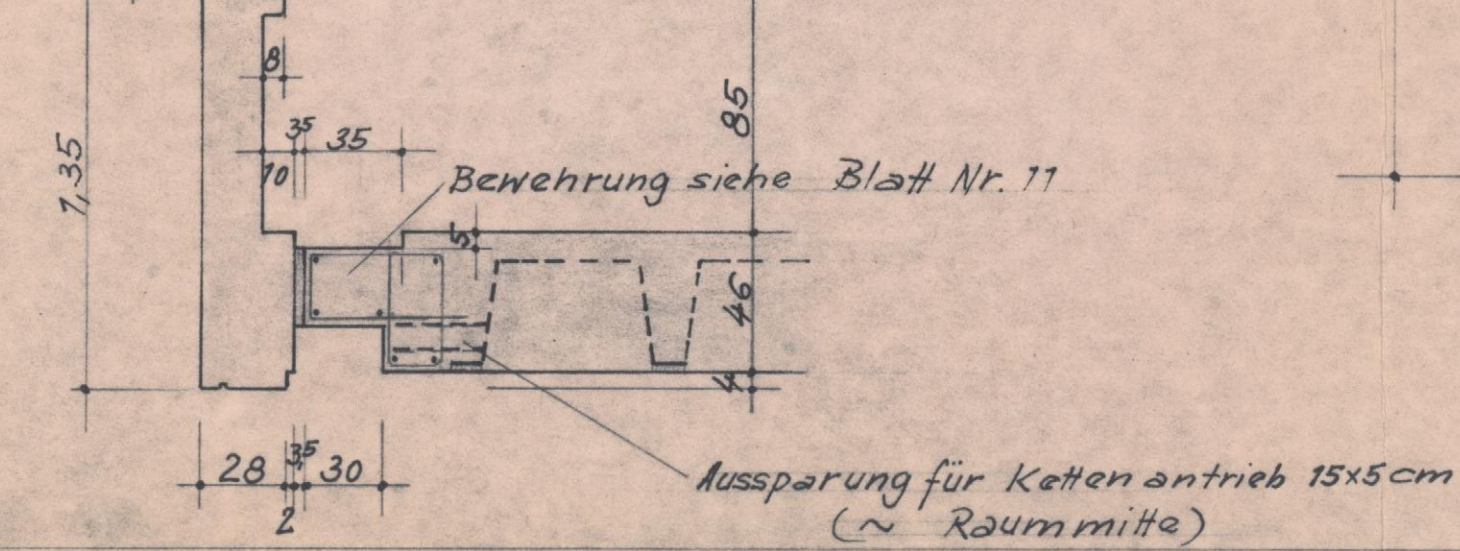
Schnitt g-g M. 1:25
