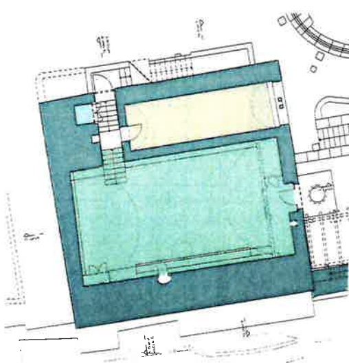
Grundriss Kellergeschoss MULTIFUNKTION | LAGER GASTRONOMIE
