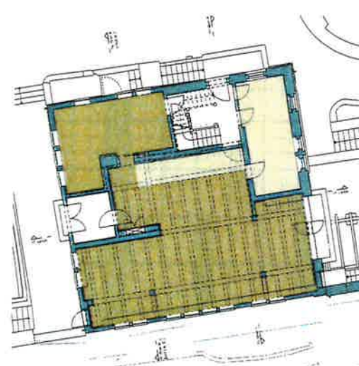
Grundriss Erdgeschoss GASTRONOMIE
