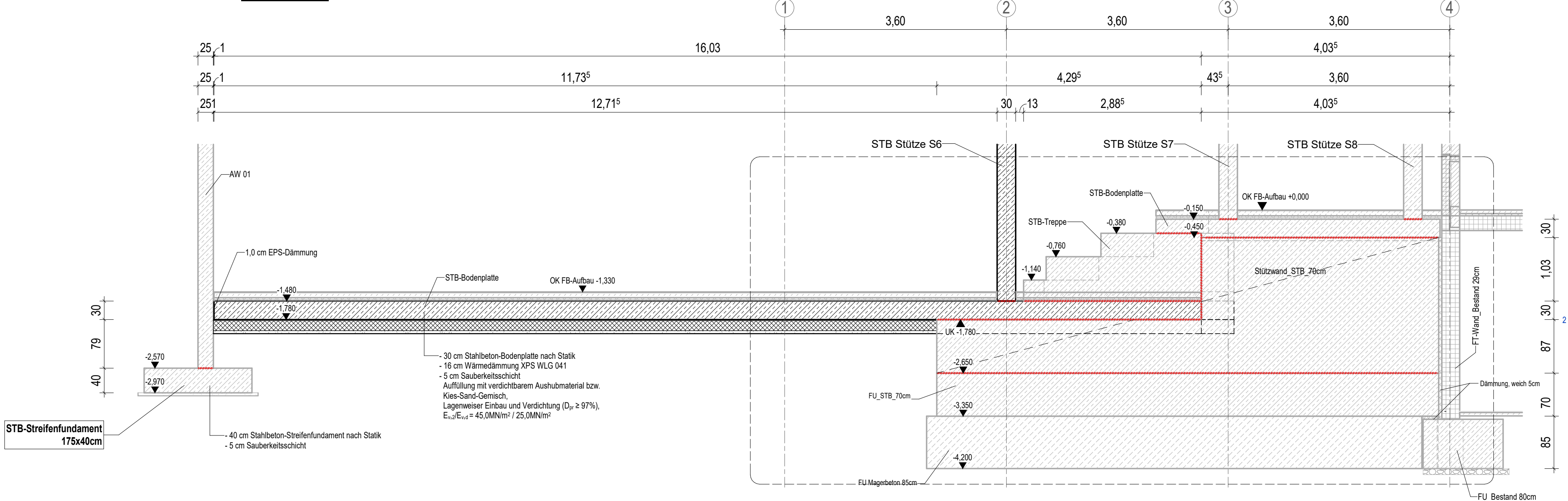
Schnitt A-A
