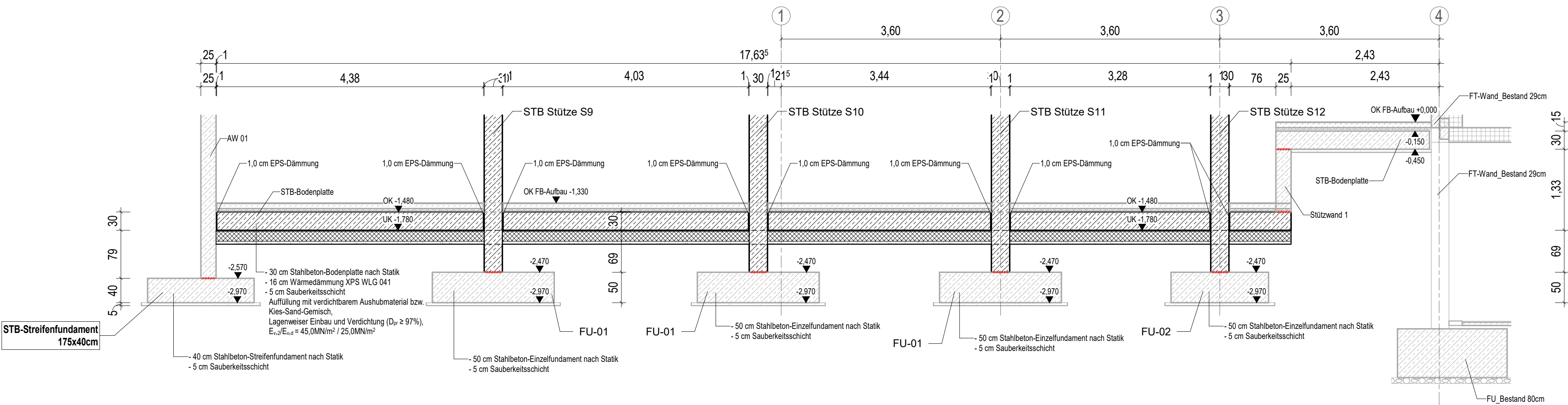
Schnitt C-C
