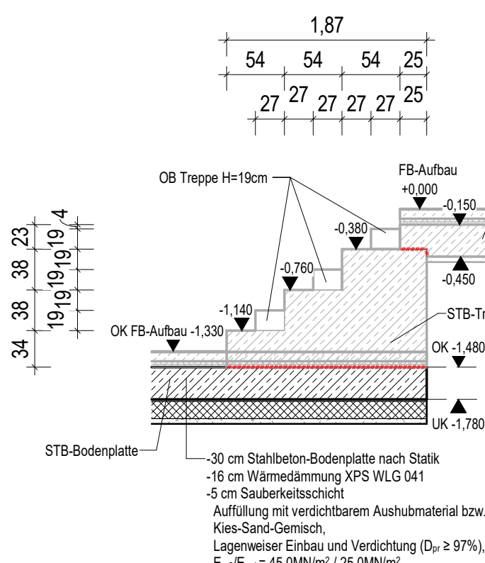
Schnitt 5-5
