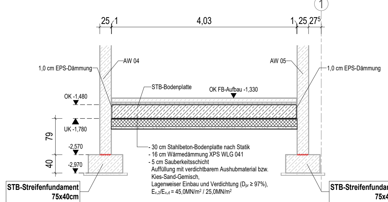
Schnitt A-A'
