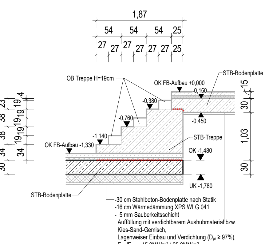
Schnitt 4-4
