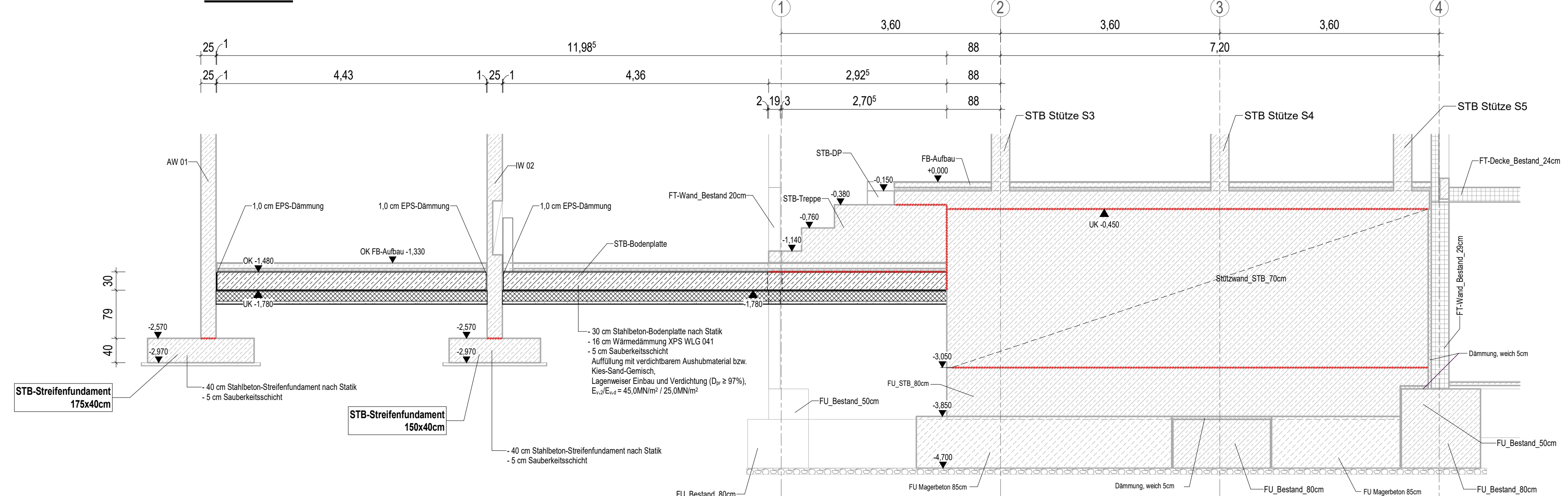
Schnitt C-C
