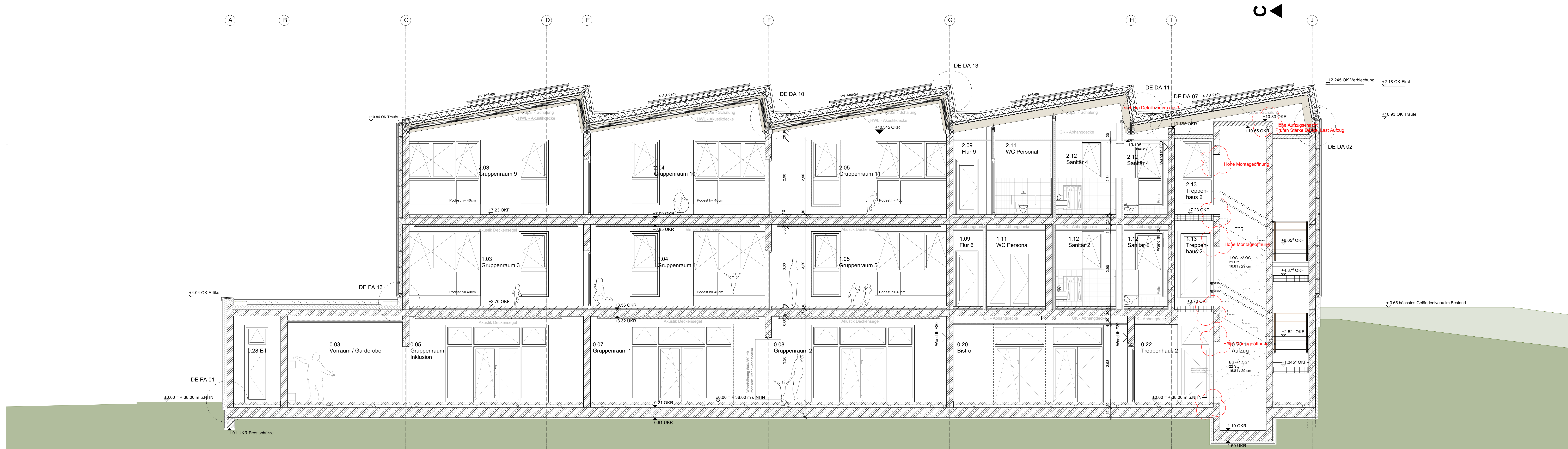
Schnitt A-A
