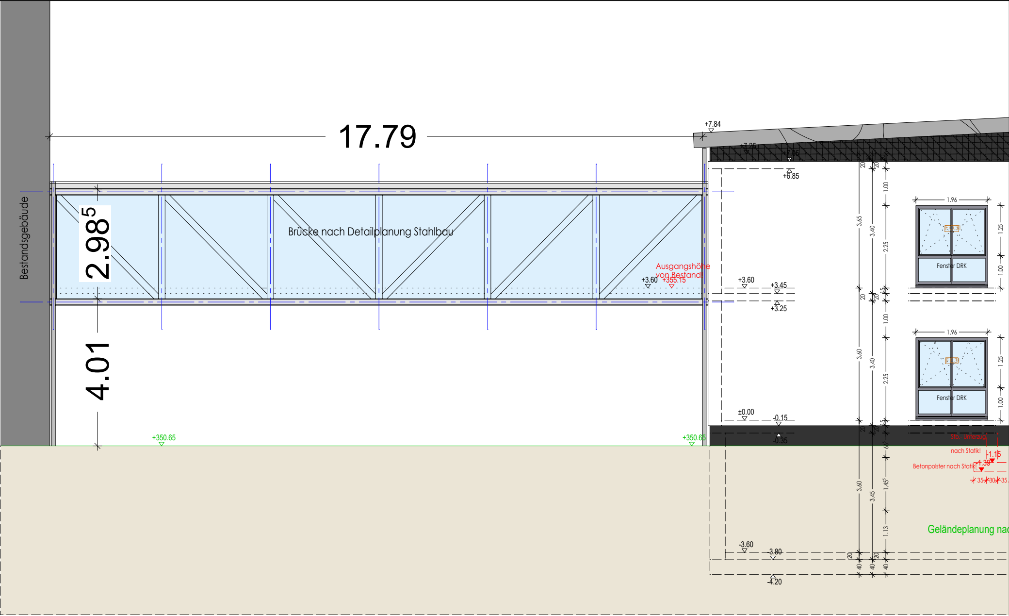
Höhenkote EG: ±0,00 = 351,55 üNN (geplant) Ansicht von Süden
