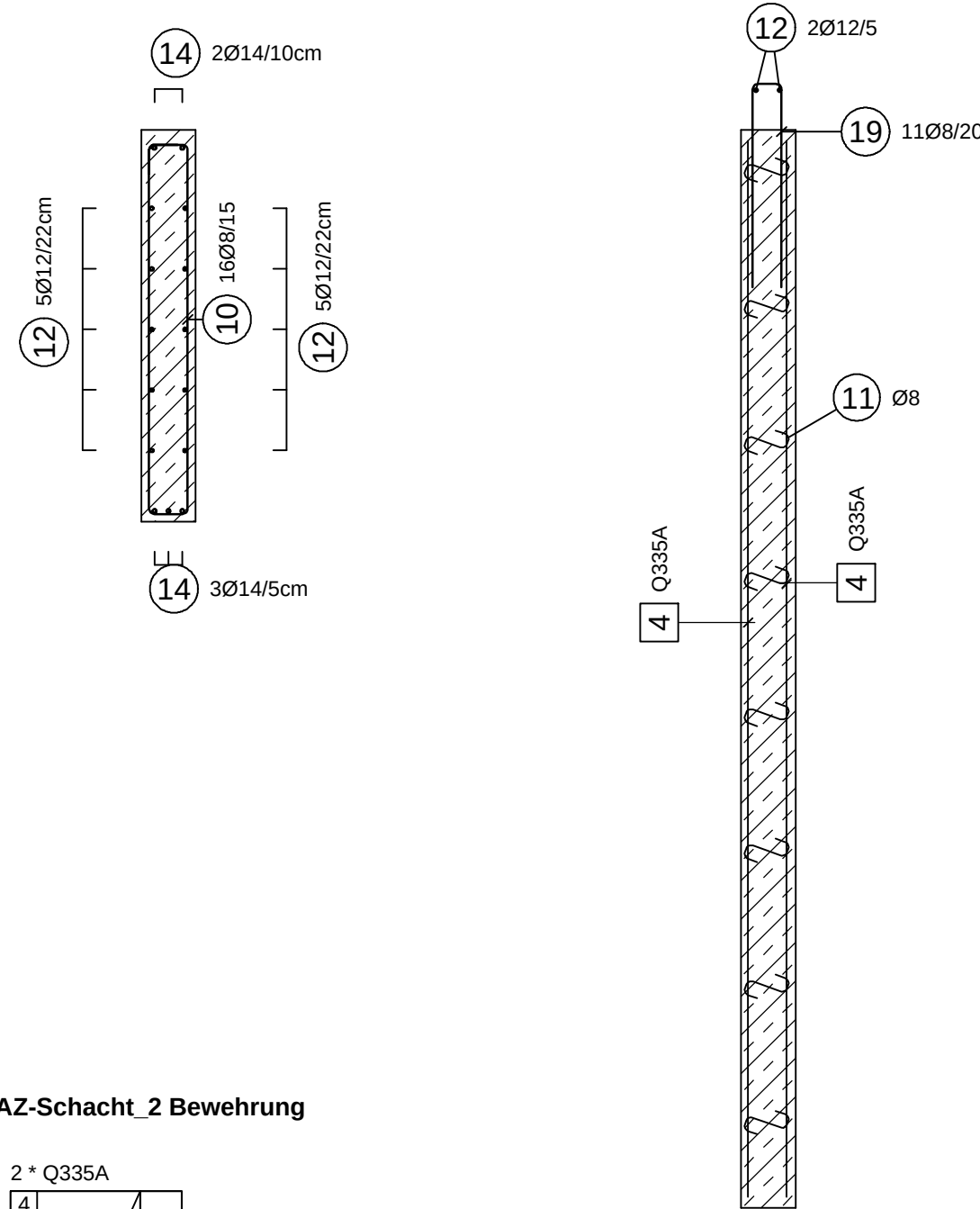
Schnitt 117 - 117
