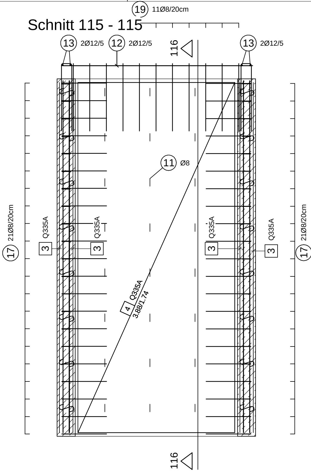
AZ-Schacht_2 Bewehrung
