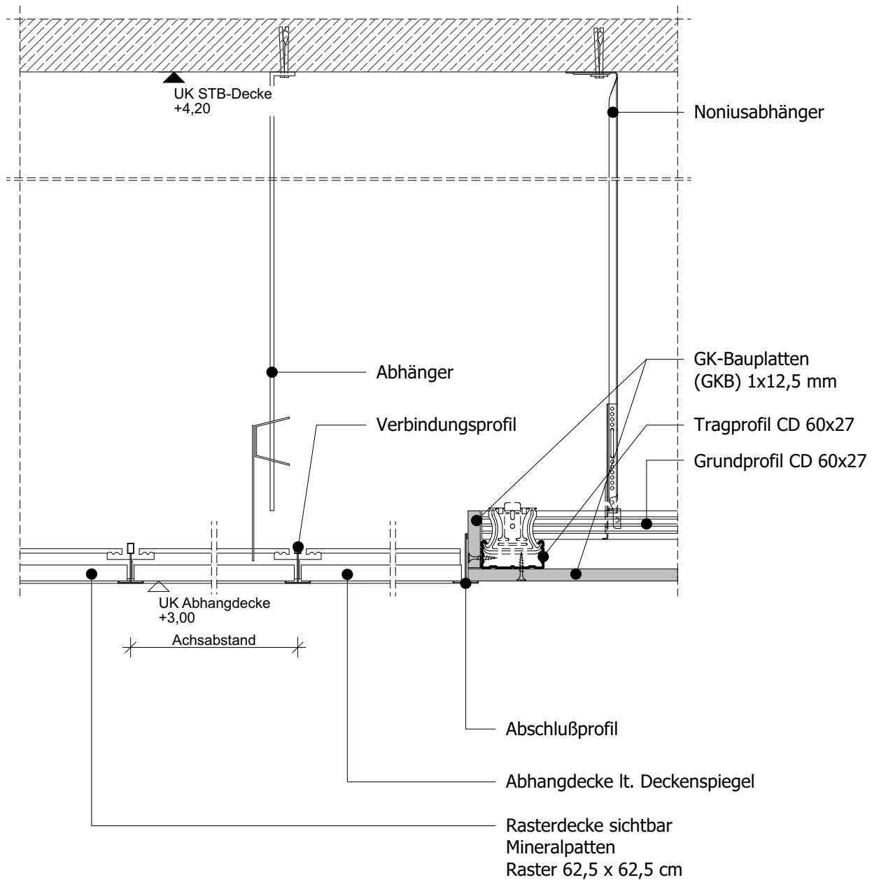
Detail Trockenbau Decke Rasterdecker / GK-Decke
