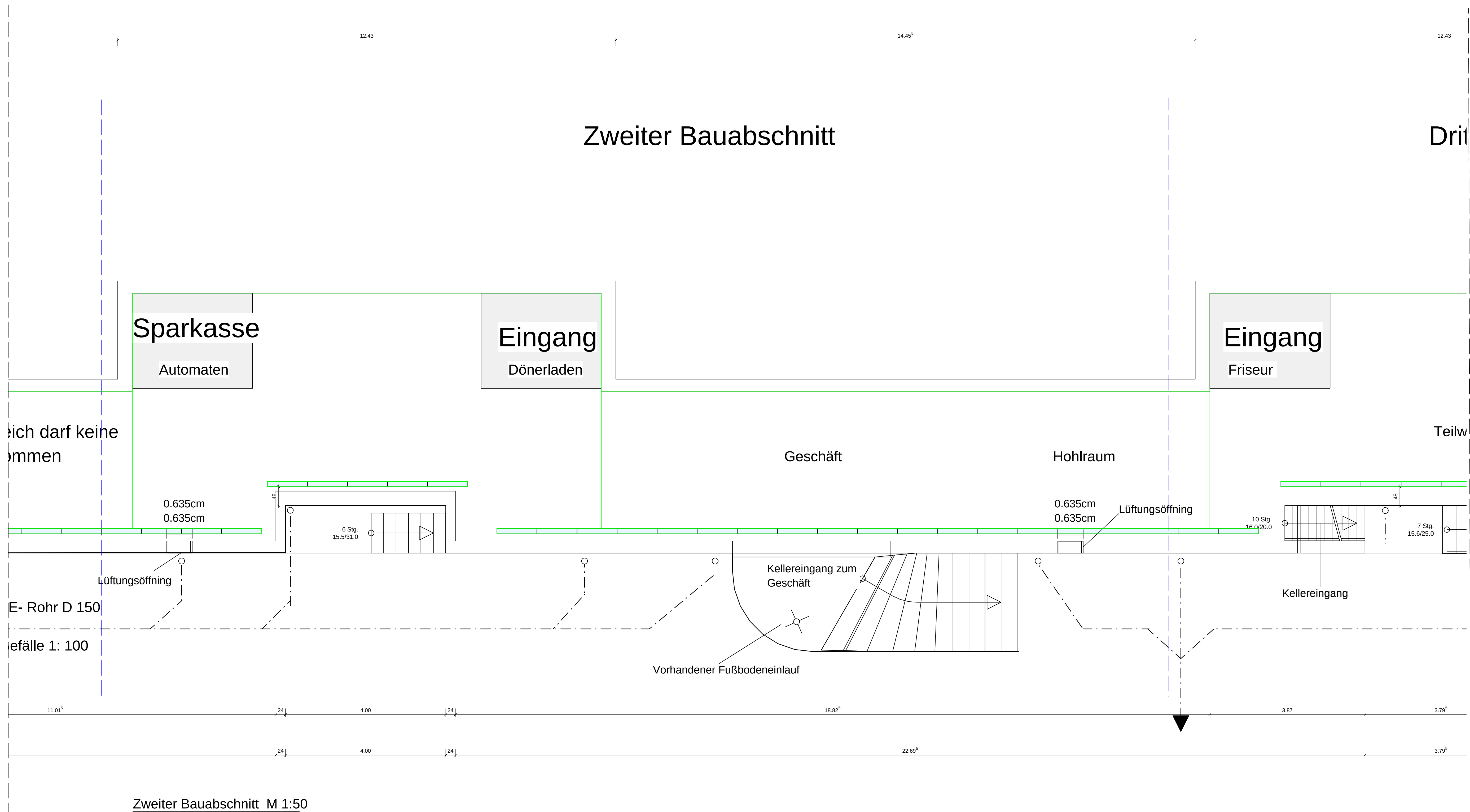
Zweiter Bauabschnitt M 1:50
