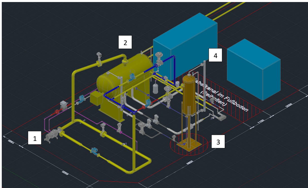
Abbildung 1: (vorläufiger) schematischer Aufbau des TP10-Demonstrators mit 1) Verdichter, 2) Dampf-/Flüssigkeitsspeicher, 3) Hochtemperatur-Speicher, 4) Schaltschränke
