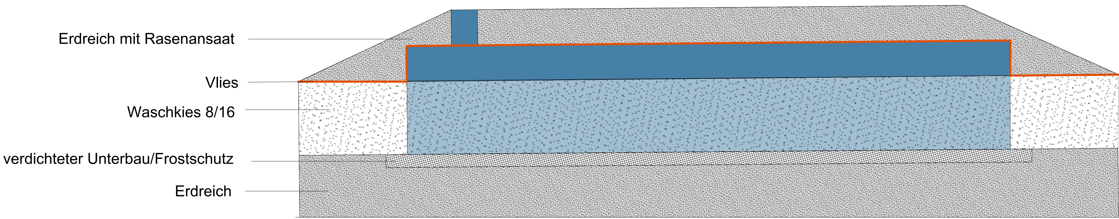
Schnitt B -BB
