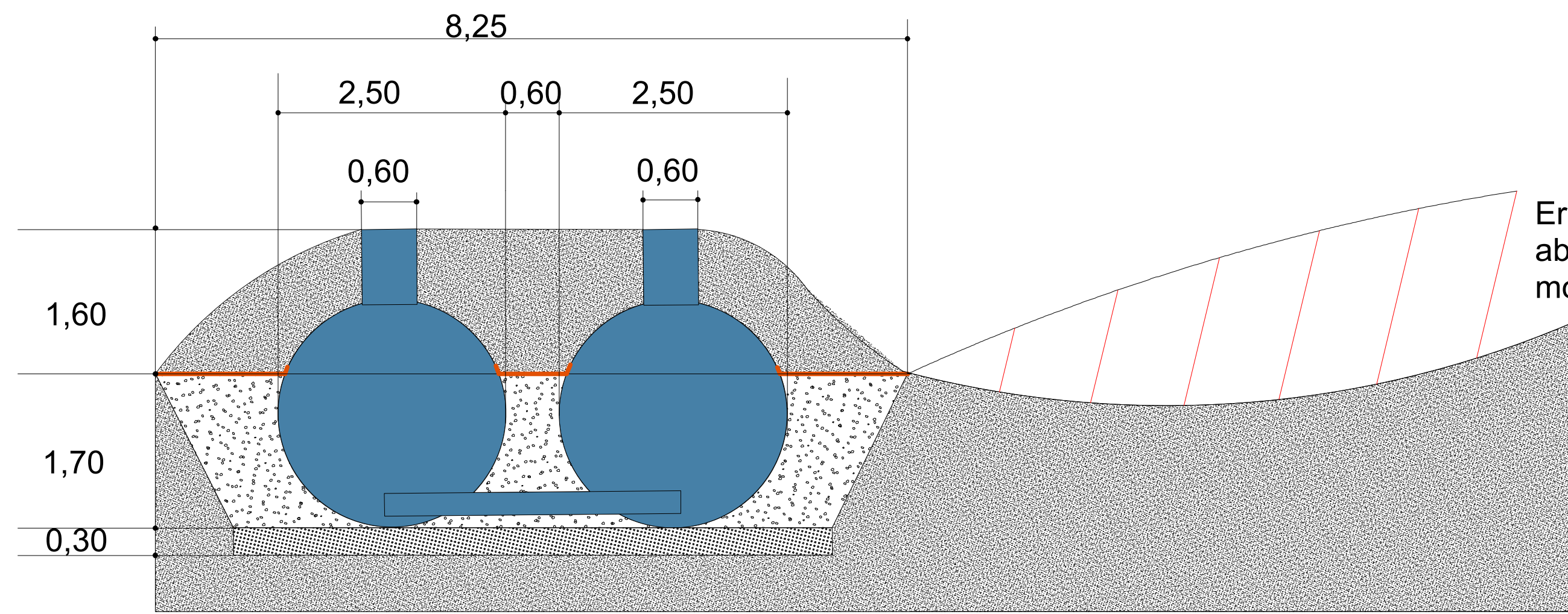
Schnitt A -AA
