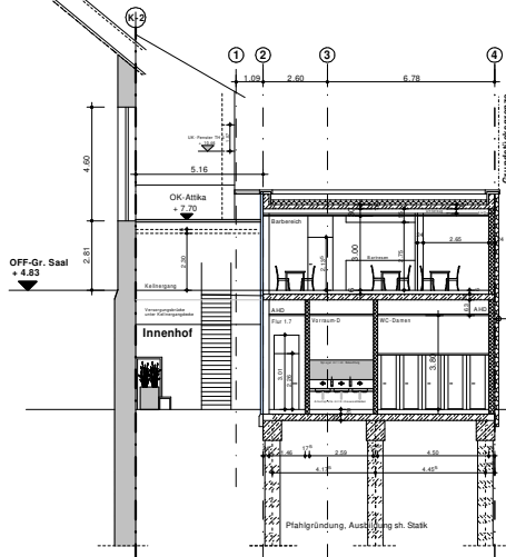
SCHNITT B - B M 1:100
