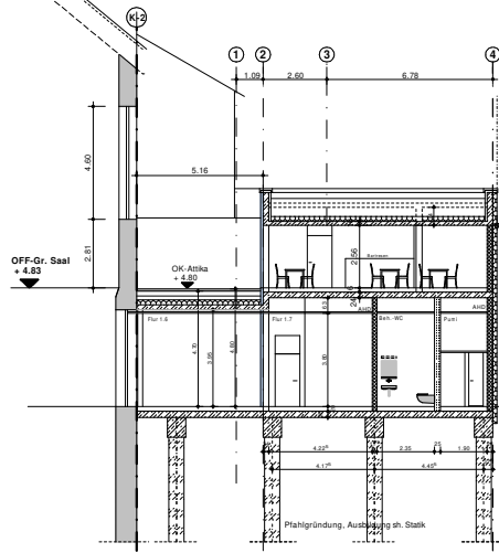
SCHNITT C - C M 1:100
