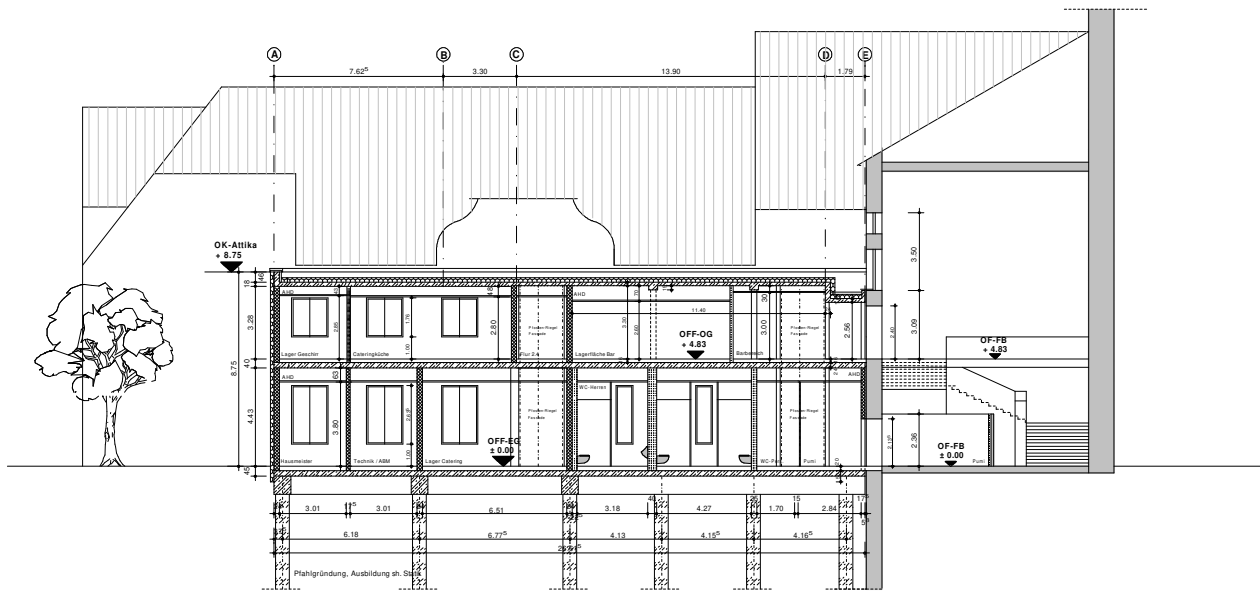
SCHNITT A - A M 1:100
