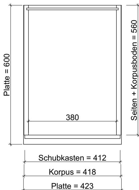
Schnitt B - B
