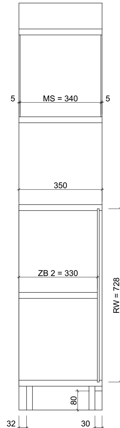
Schnitt C - C
