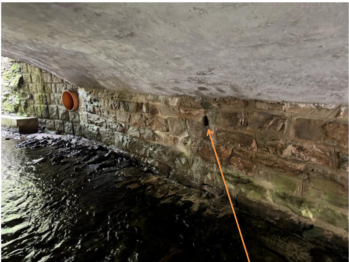
Lage Diamantkernbohrung (DKB) Nr. I
