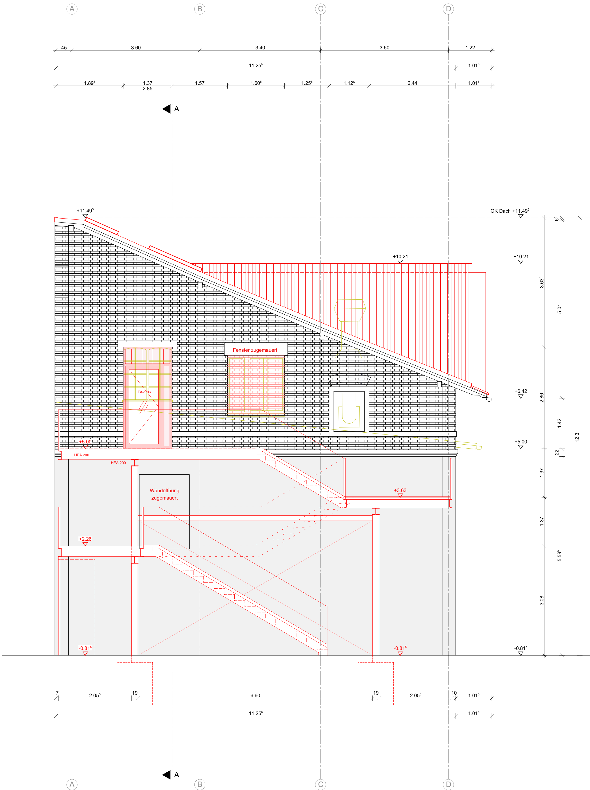
Ansicht Süd
