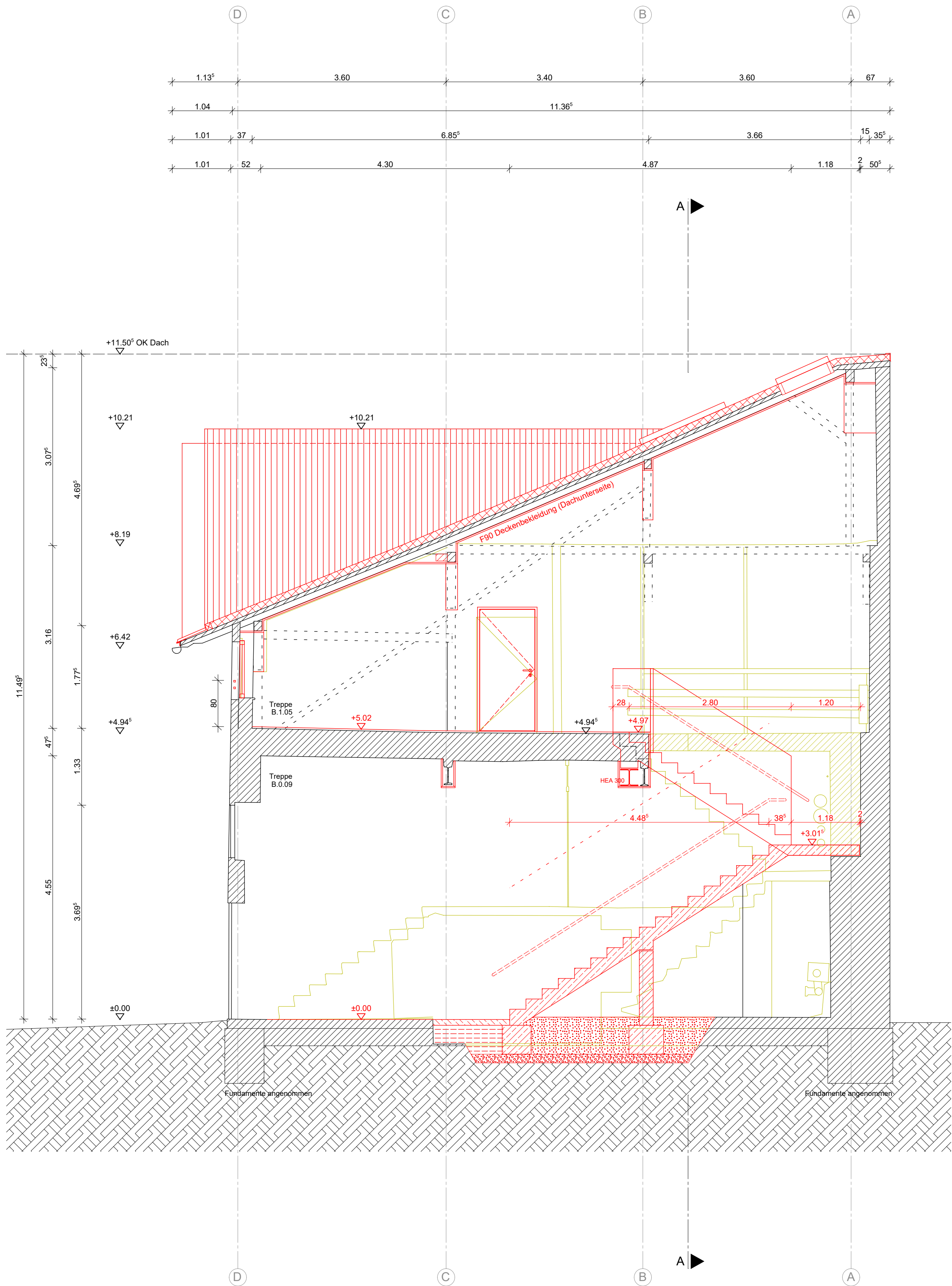
Schnitt B - B
