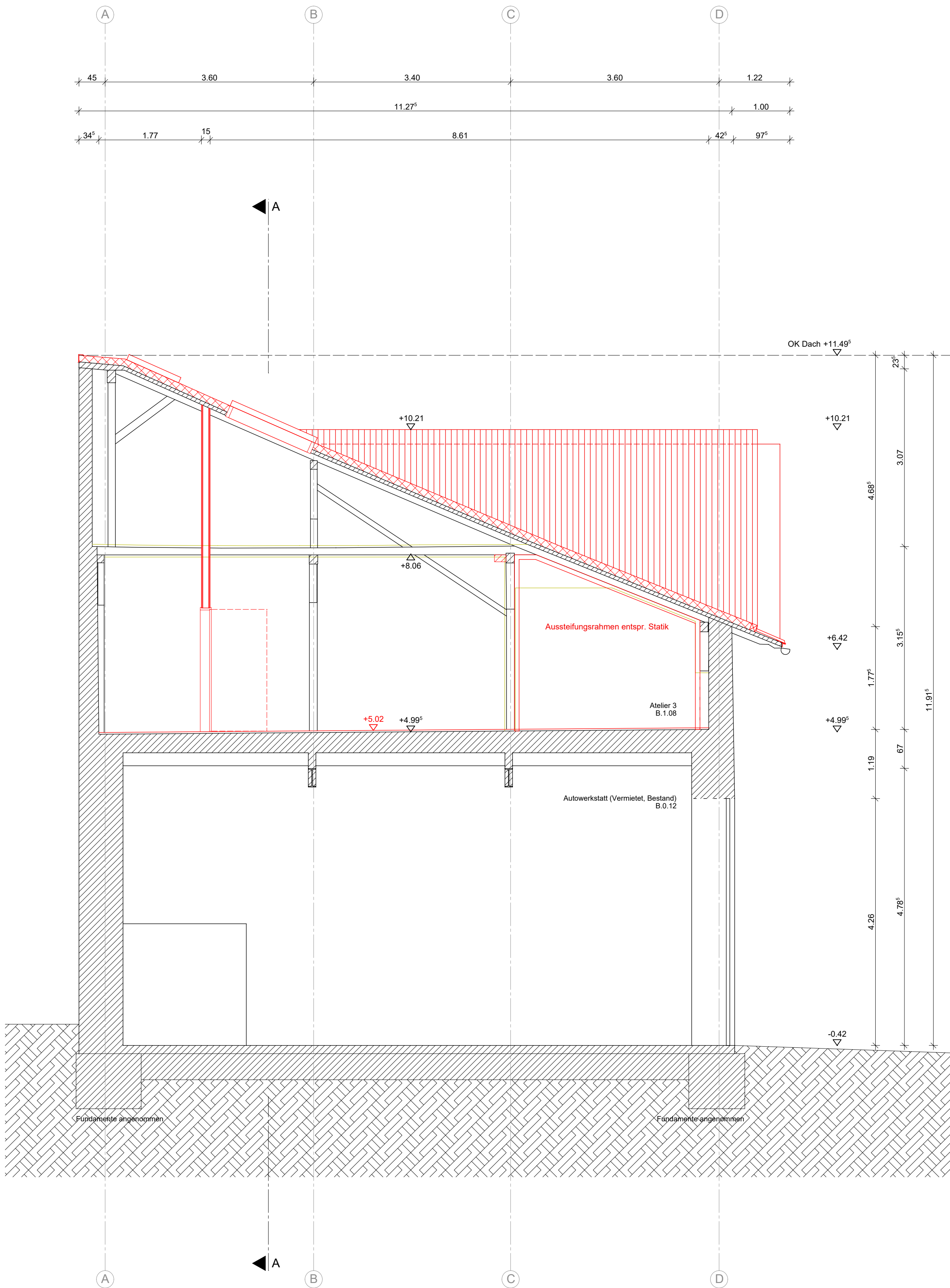
Schnitt C - C
