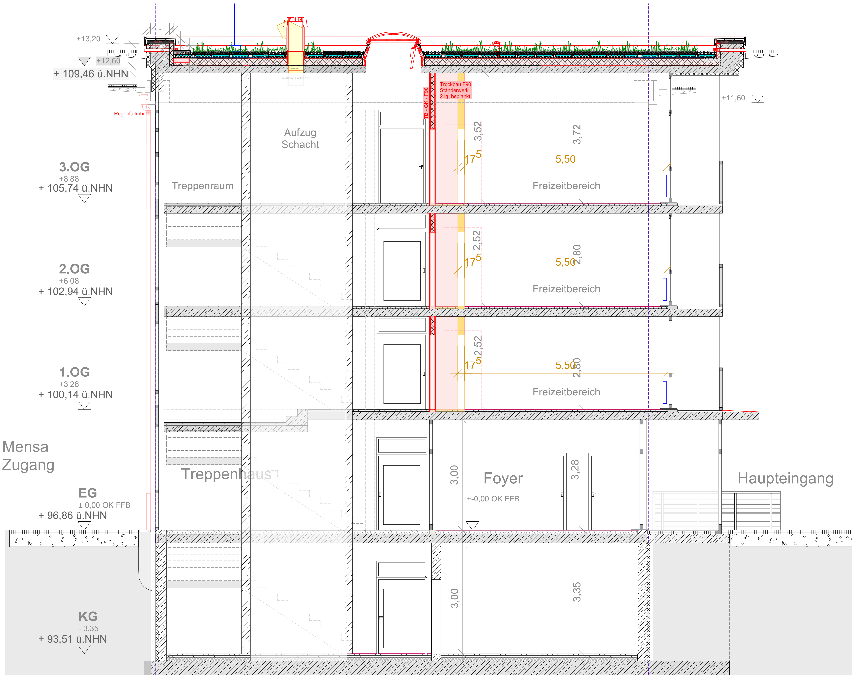
Schnitt B-B
