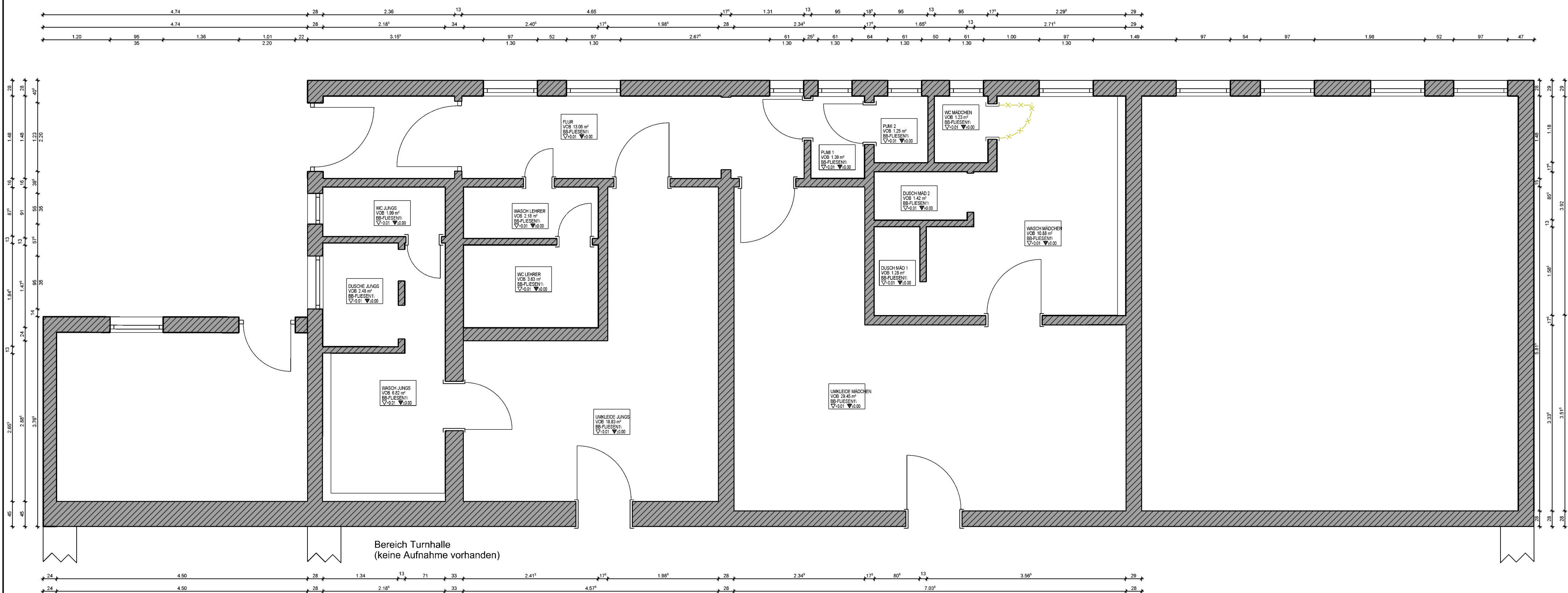
Erdgeschoß BAU Bestand
