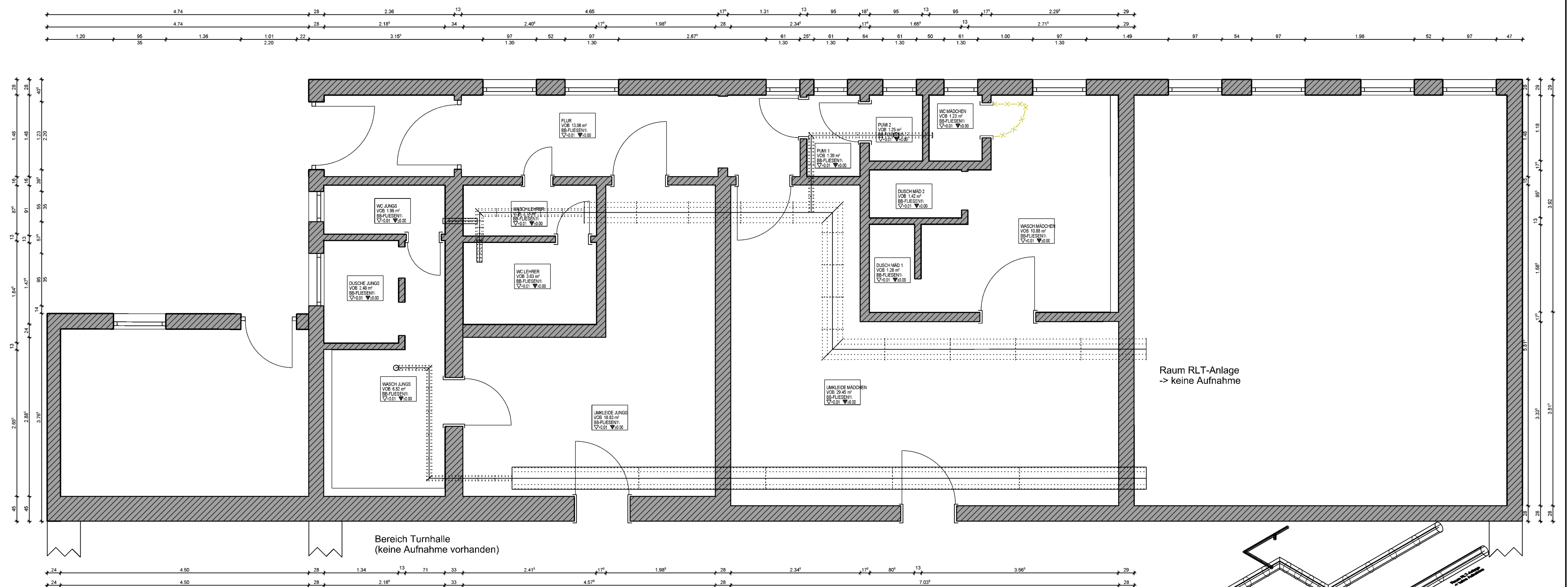
Erdgeschoß LÜFTUNG Bestand
