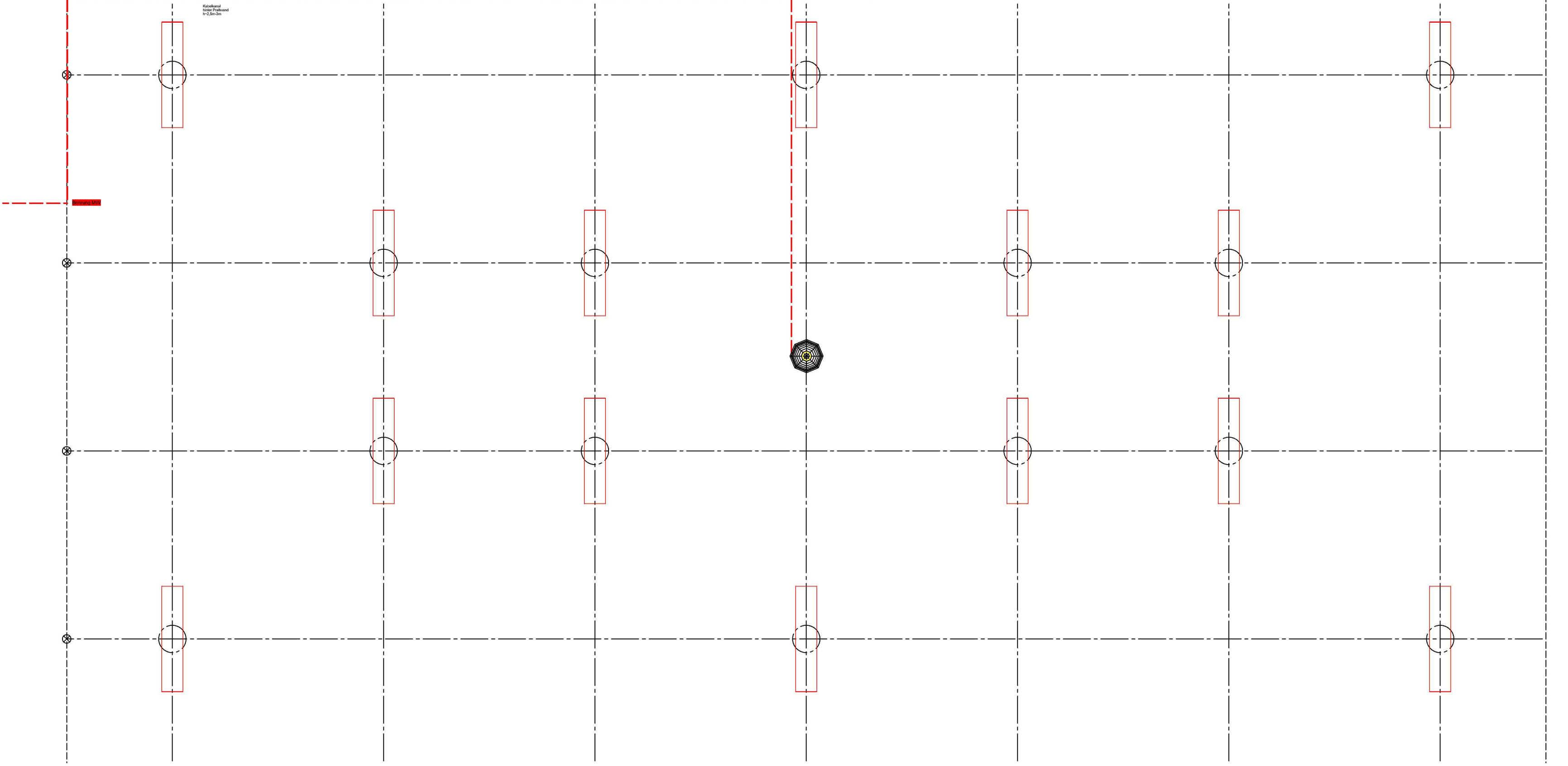
Erdgeschoß ELEKTRO Neubau
