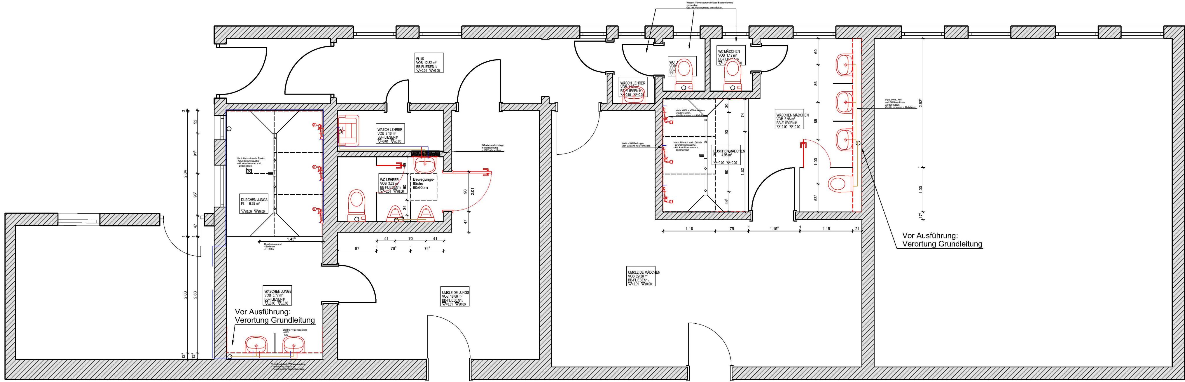
Erdgeschoß SANITÄR Neubau
