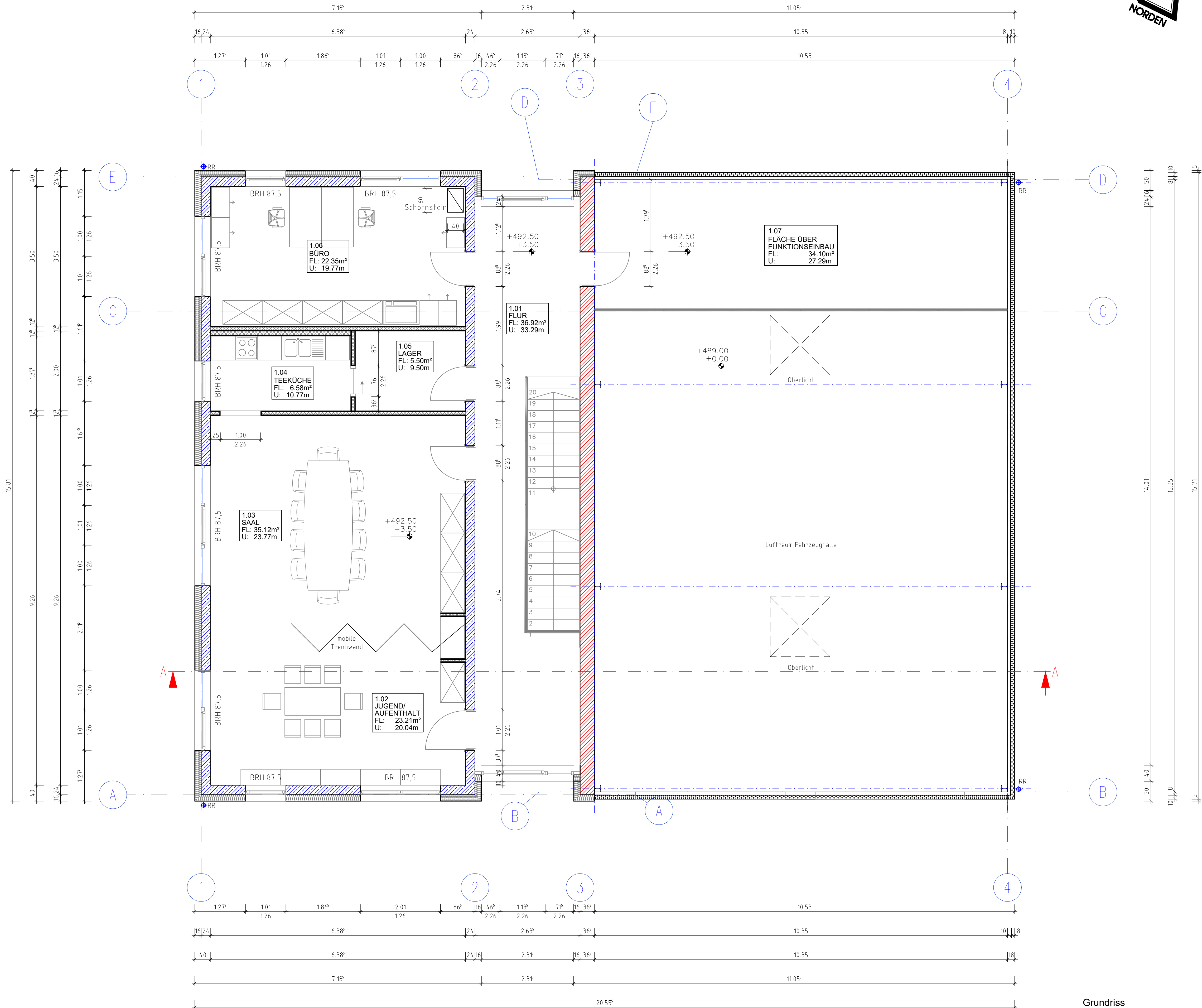
Grundriss Obergeschoss
