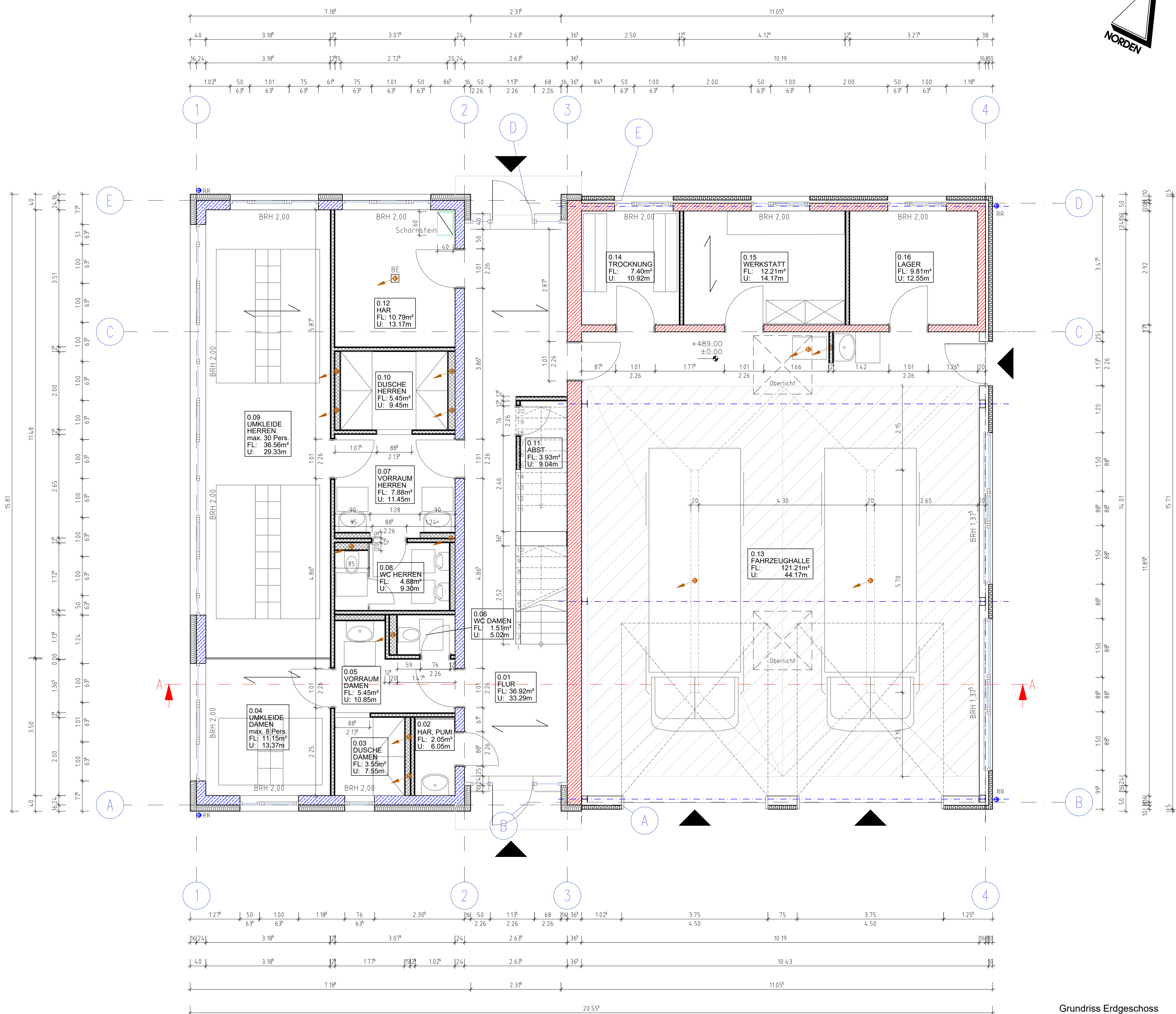
Grundriss Erdgeschoss
