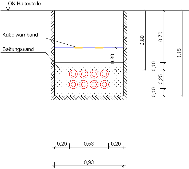
Querschnitt 19
