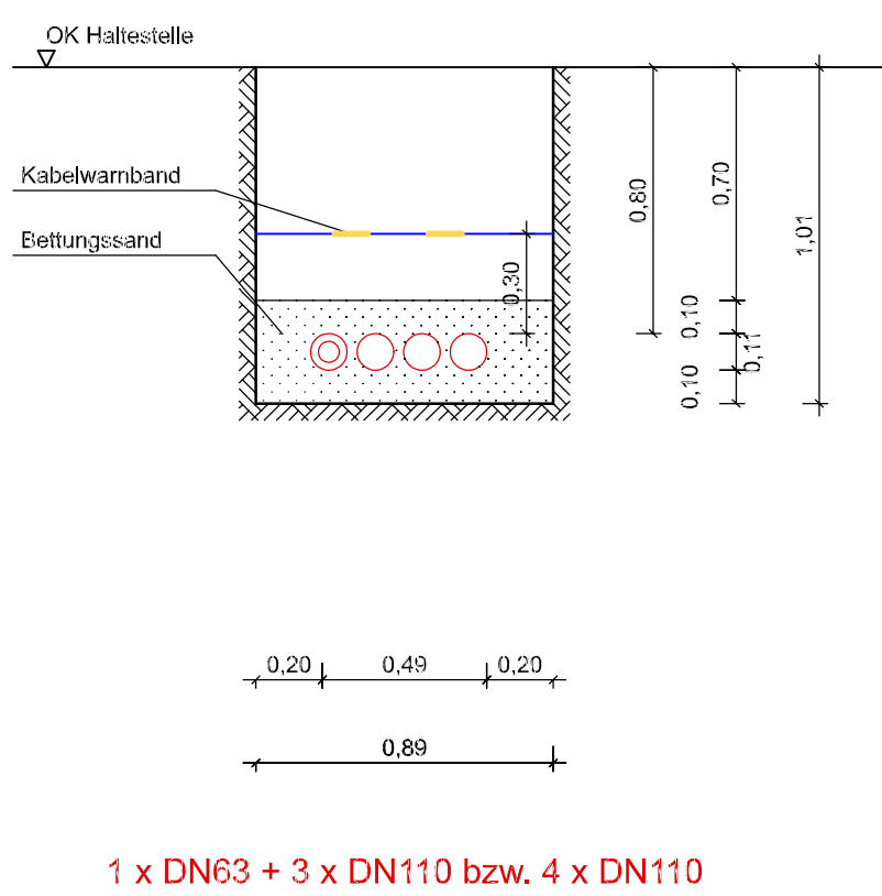
Querschnitt 14
