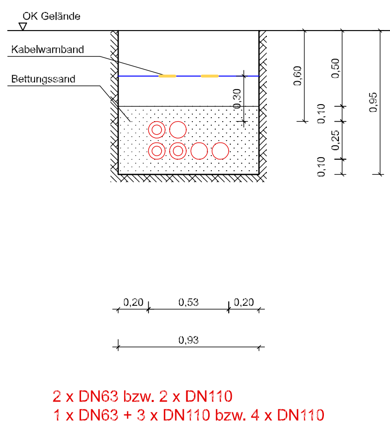
Querschnitt 13
