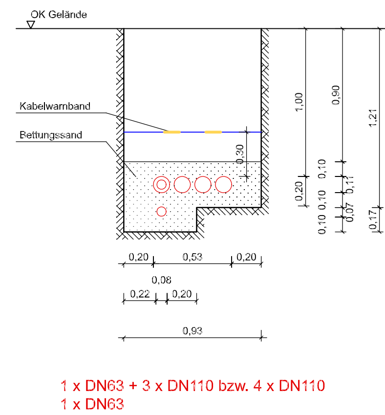
Querschnitt 11
