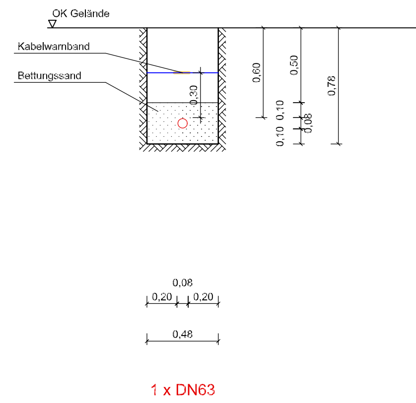
Querschnitt 6
