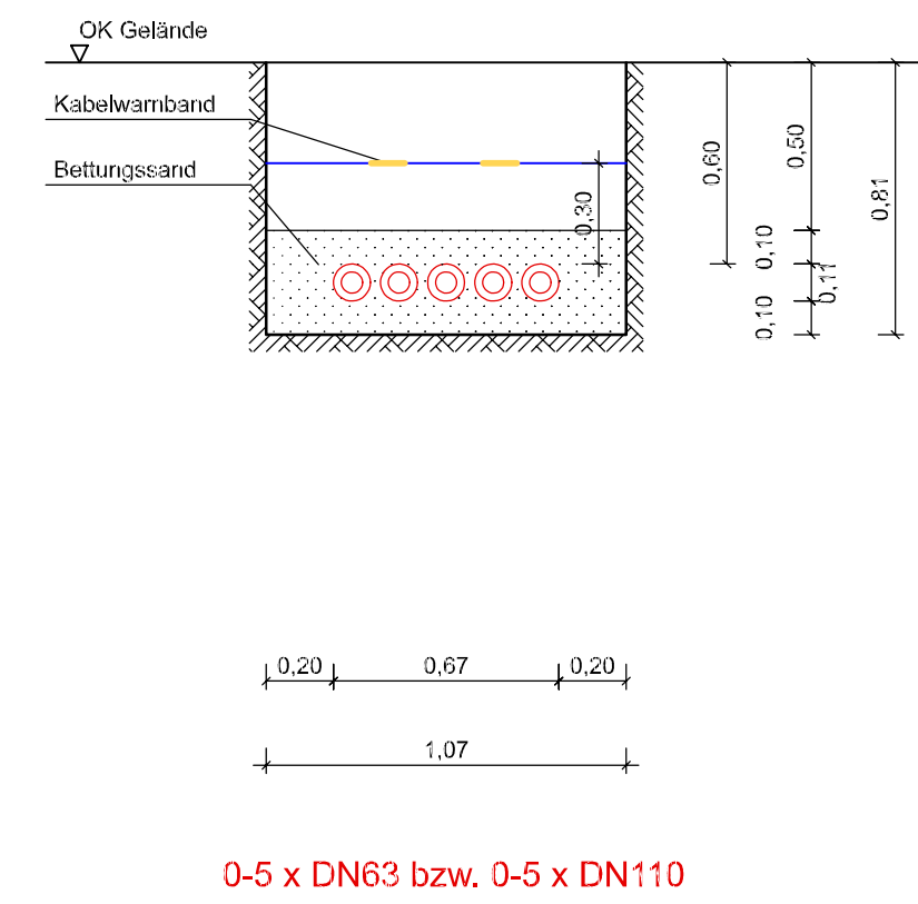
Querschnitt 8
