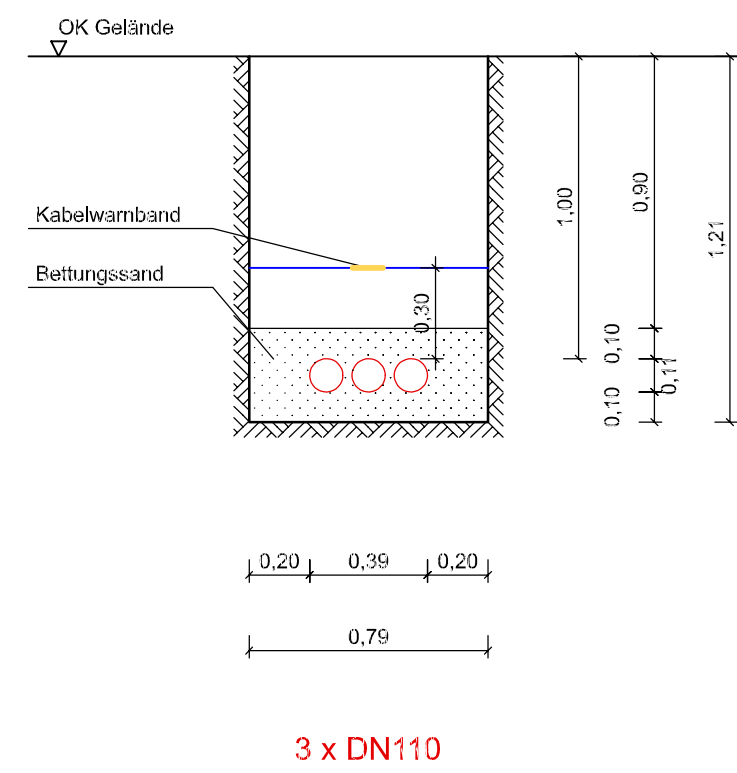
Querschnitt 2
