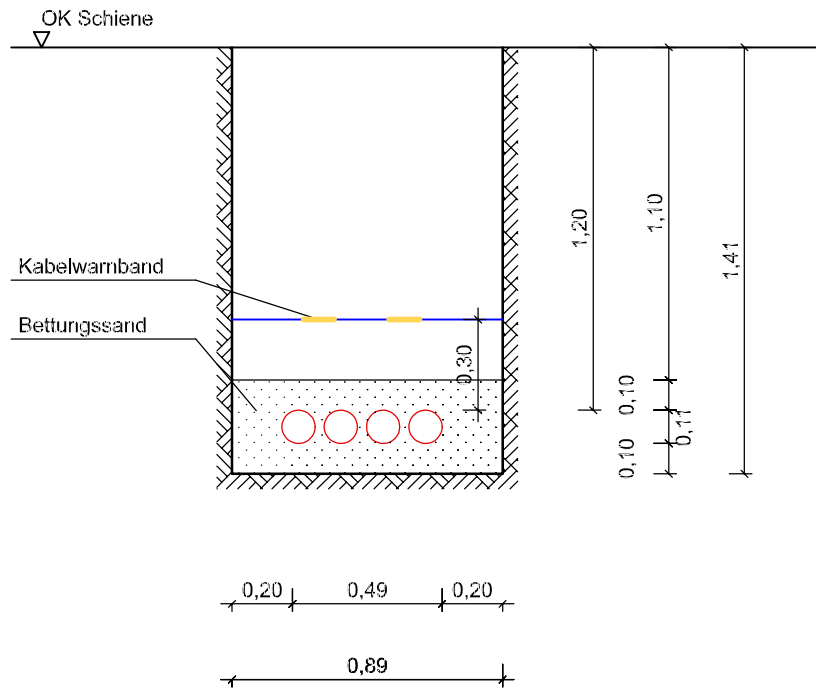
Querschnitt 24
