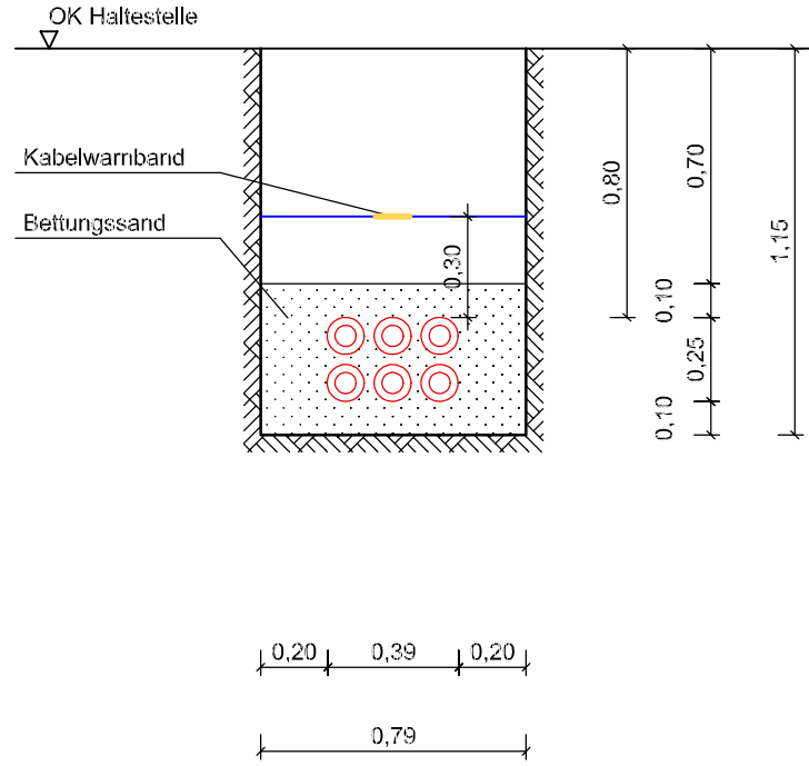
Querschnitt 20
