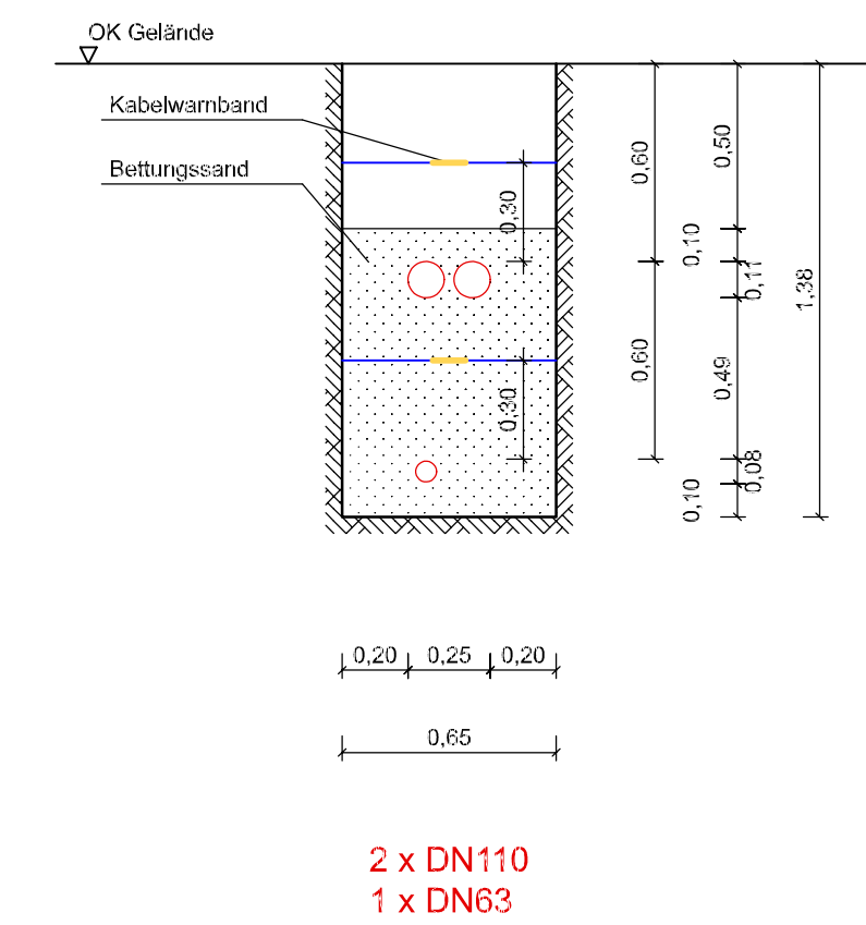
Querschnitt 12
