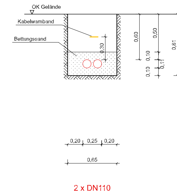
Querschnitt 4
