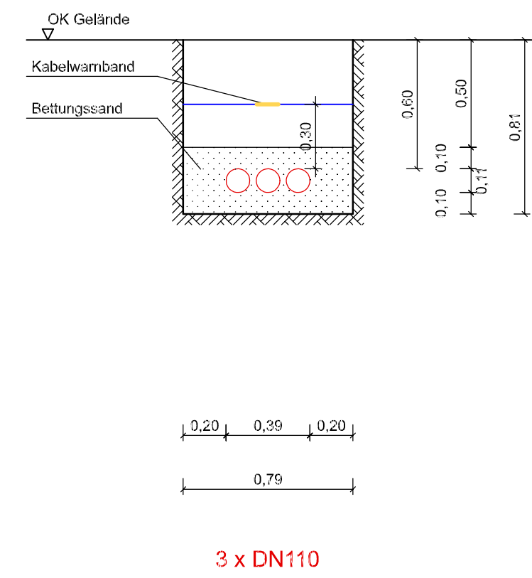
Querschnitt 5
