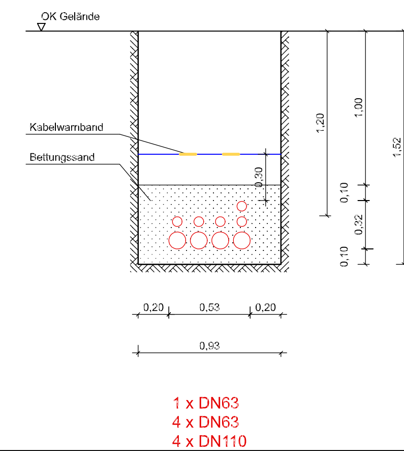
Querschnitt 16
