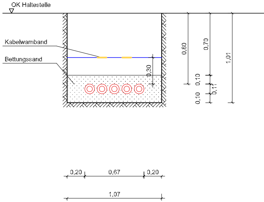
Querschnitt 25
