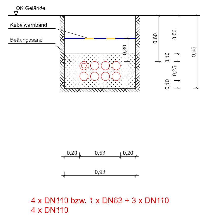
Querschnitt 15
