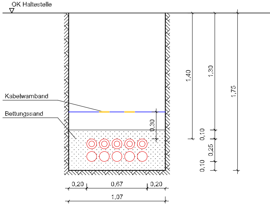
Querschnitt 17
