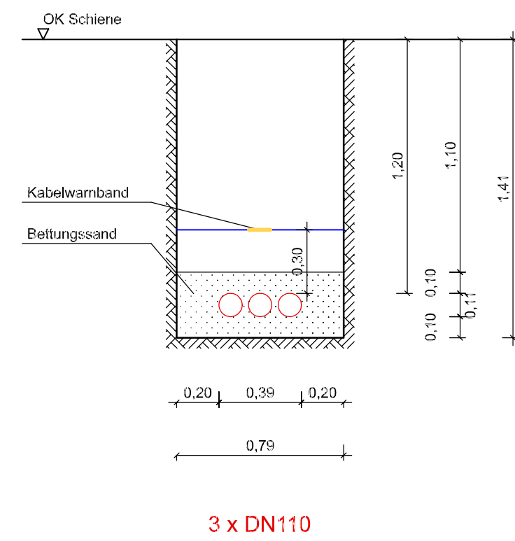
Querschnitt 3
