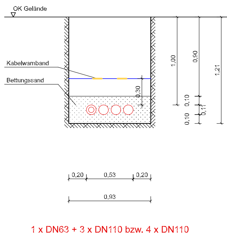
Querschnitt 9
