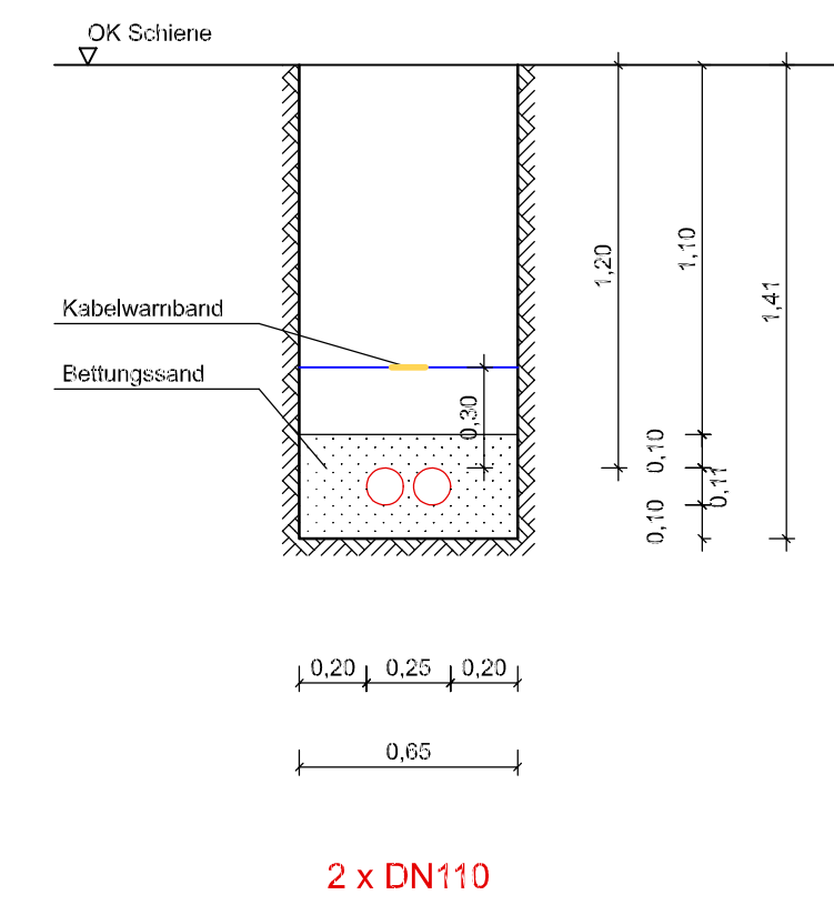
Querschnitt 10
