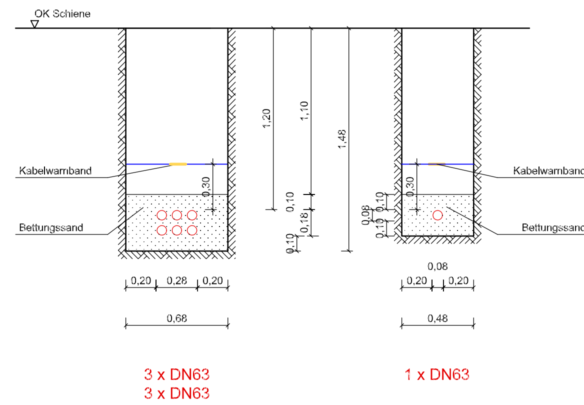
Querschnitt 1
