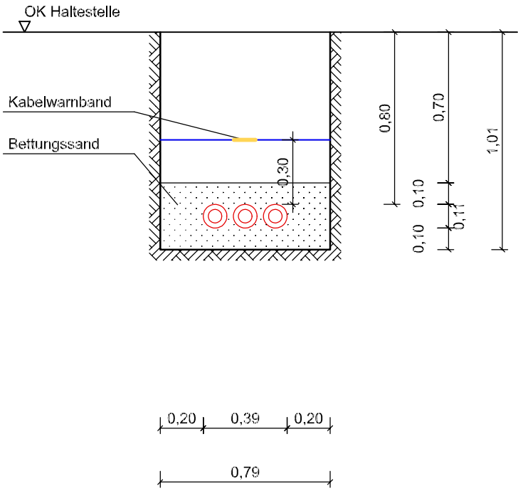
Querschnitt 26
