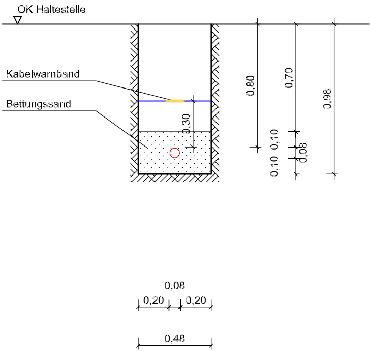
Querschnitt 22
