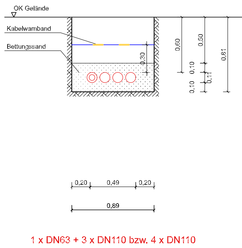
Querschnitt 7
