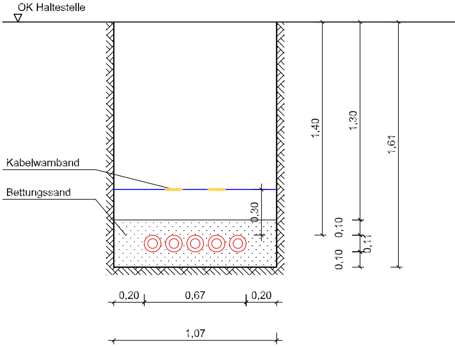
Querschnitt 18
