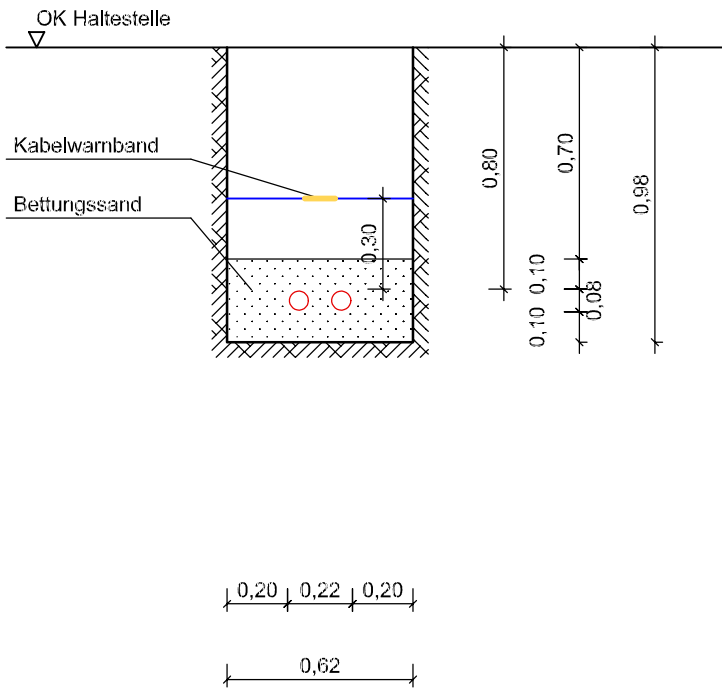
Querschnitt 23
