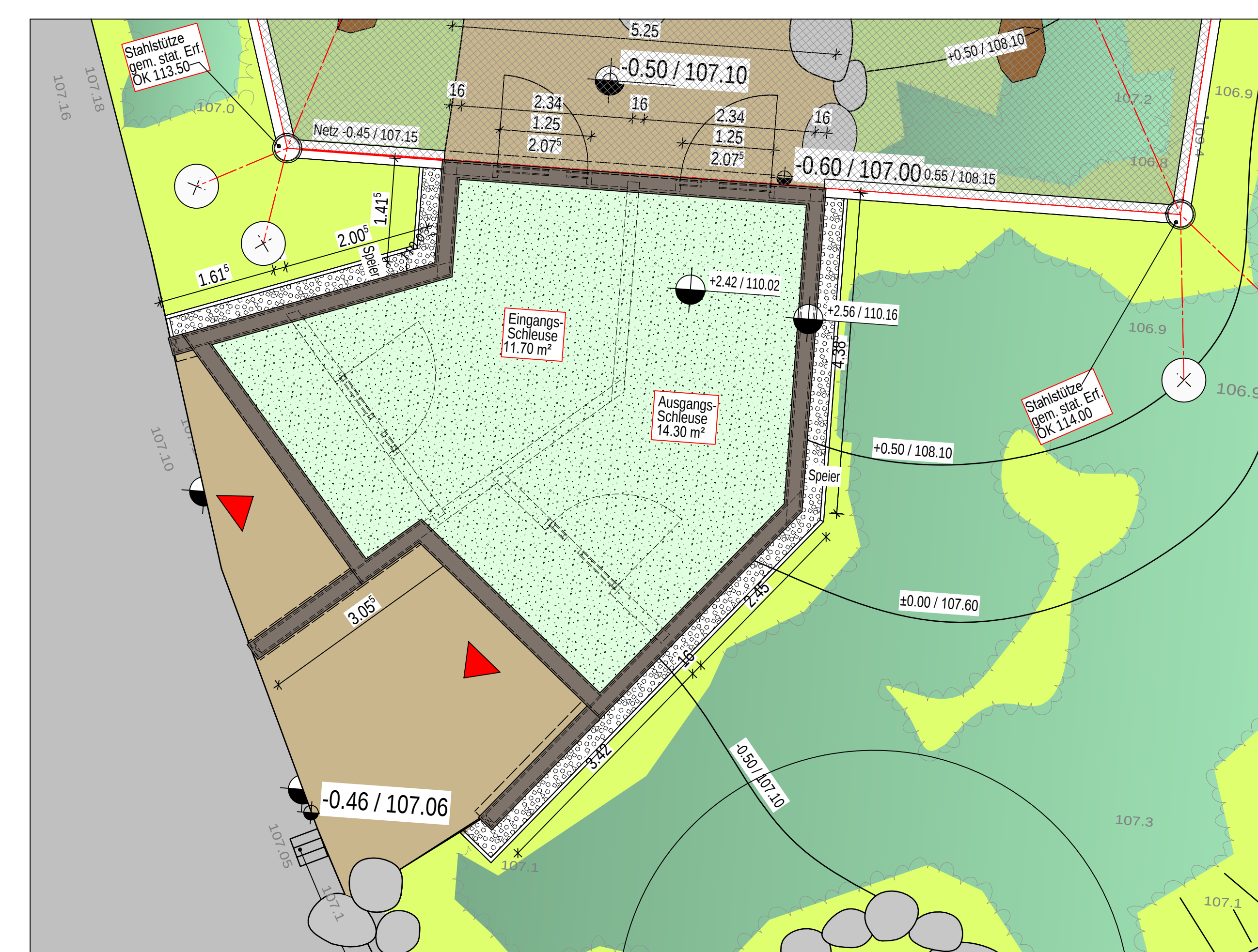
Dachaufsicht 1:50
