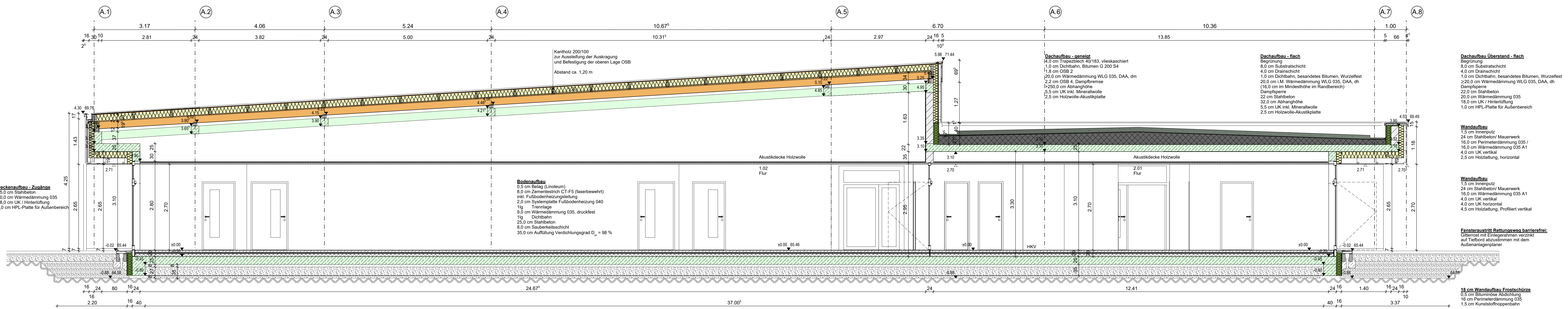
Schnitt D-D
