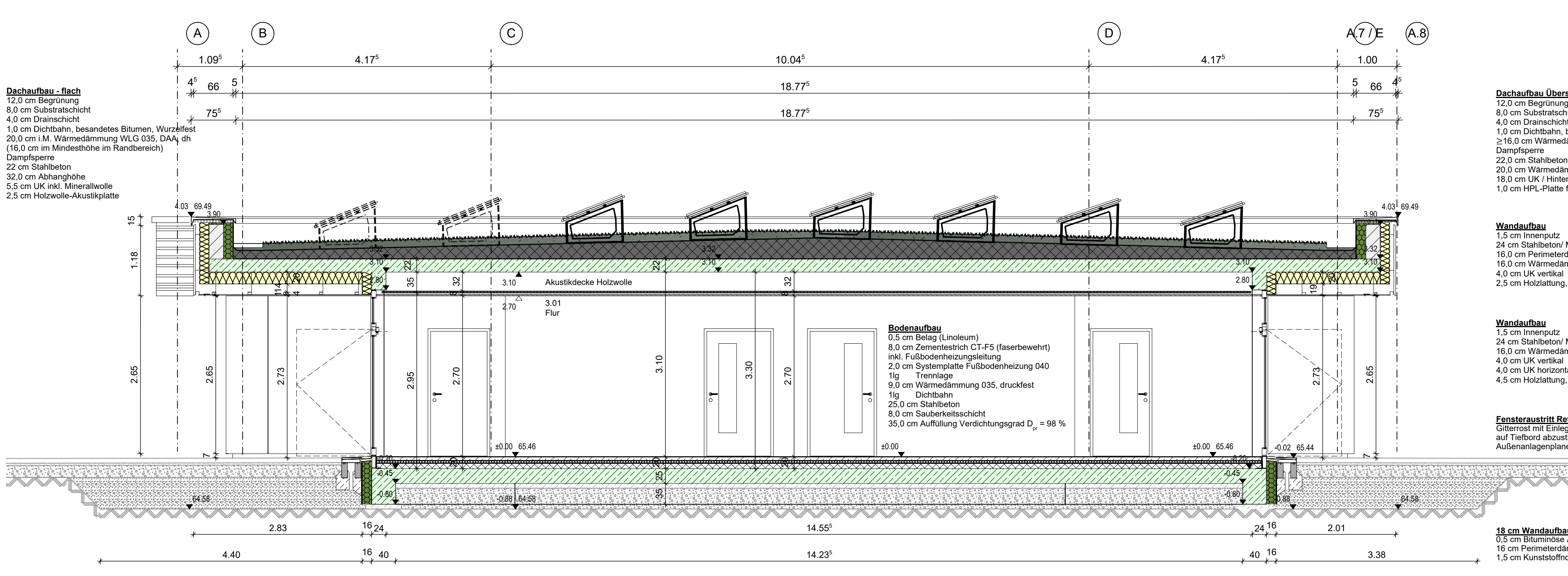
Schnitt F-F
