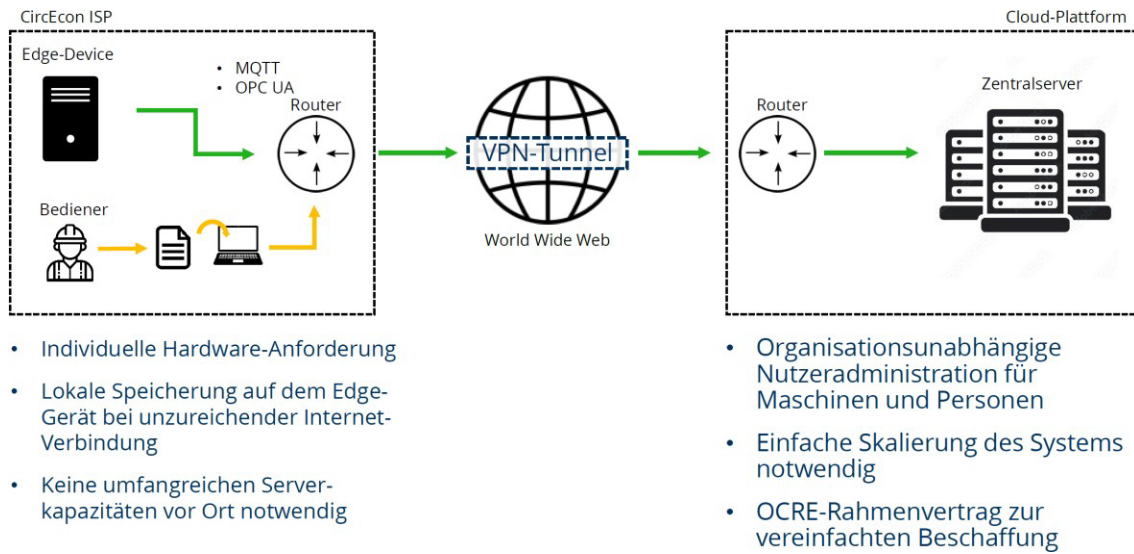
Abbildung 13: Web-basierte Netzwerkarchitektur (Quelle : ILK TU Dresden)
