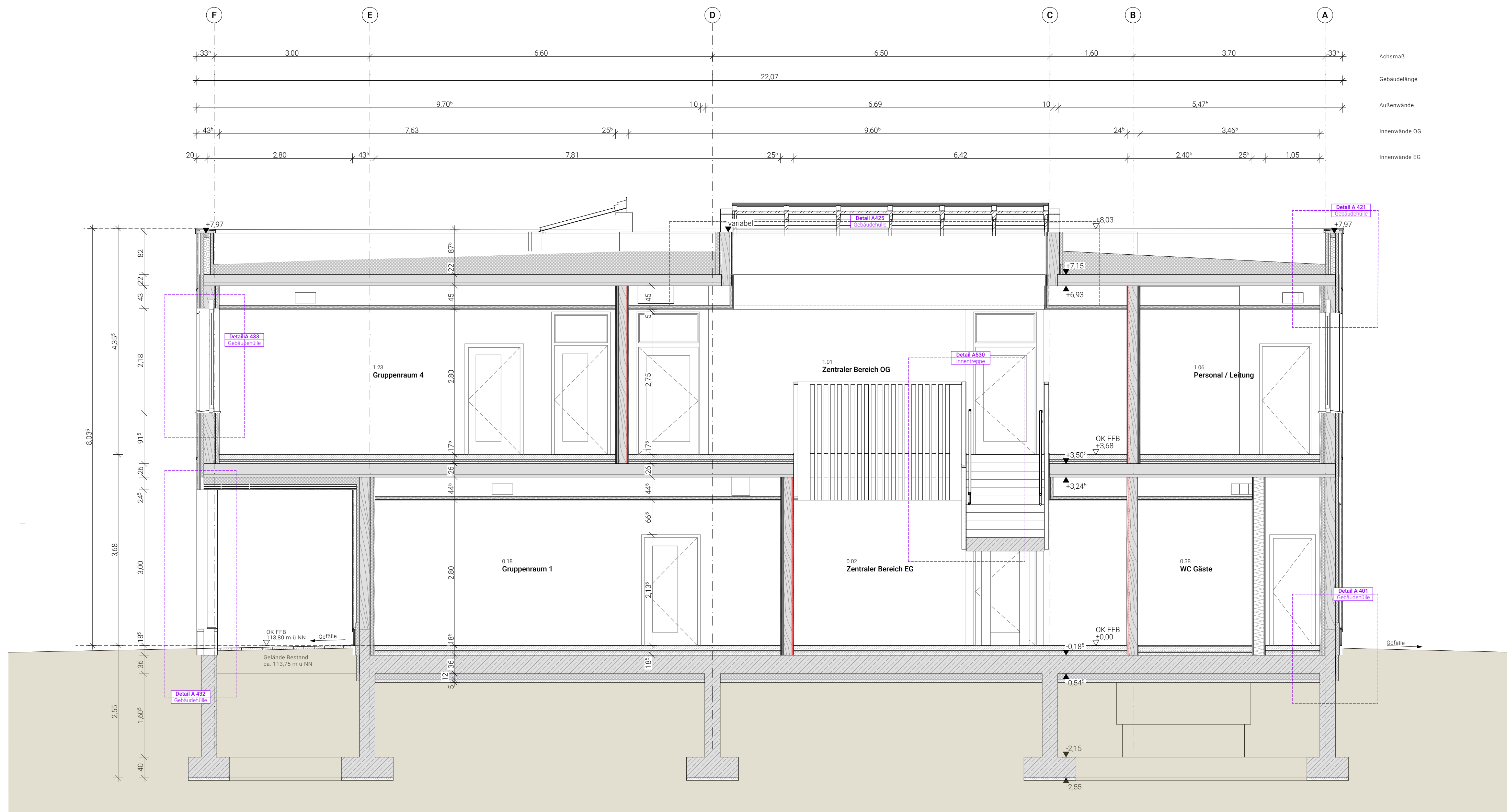
Querschnitt B-B
