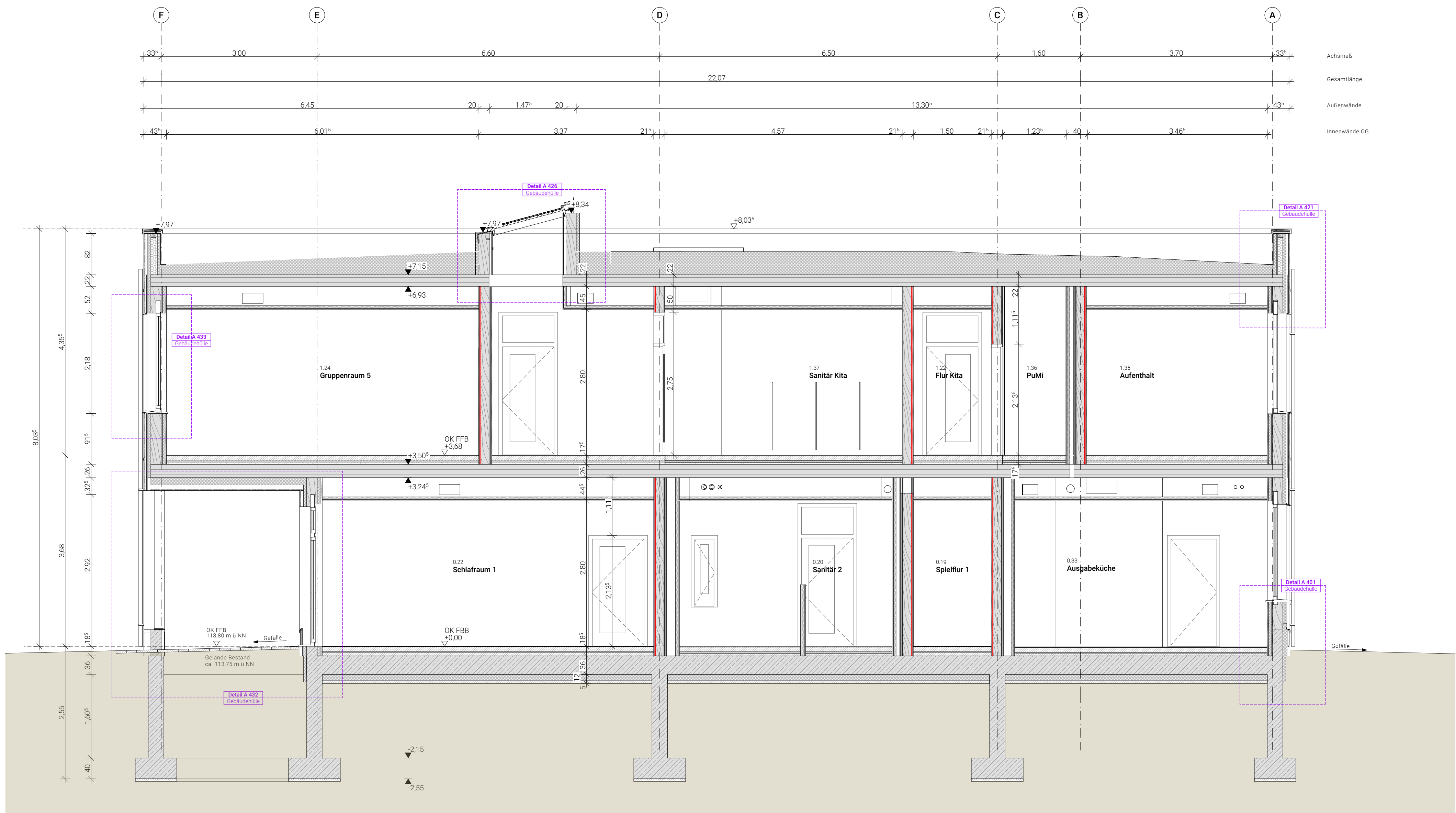
Querschnitt C-C
