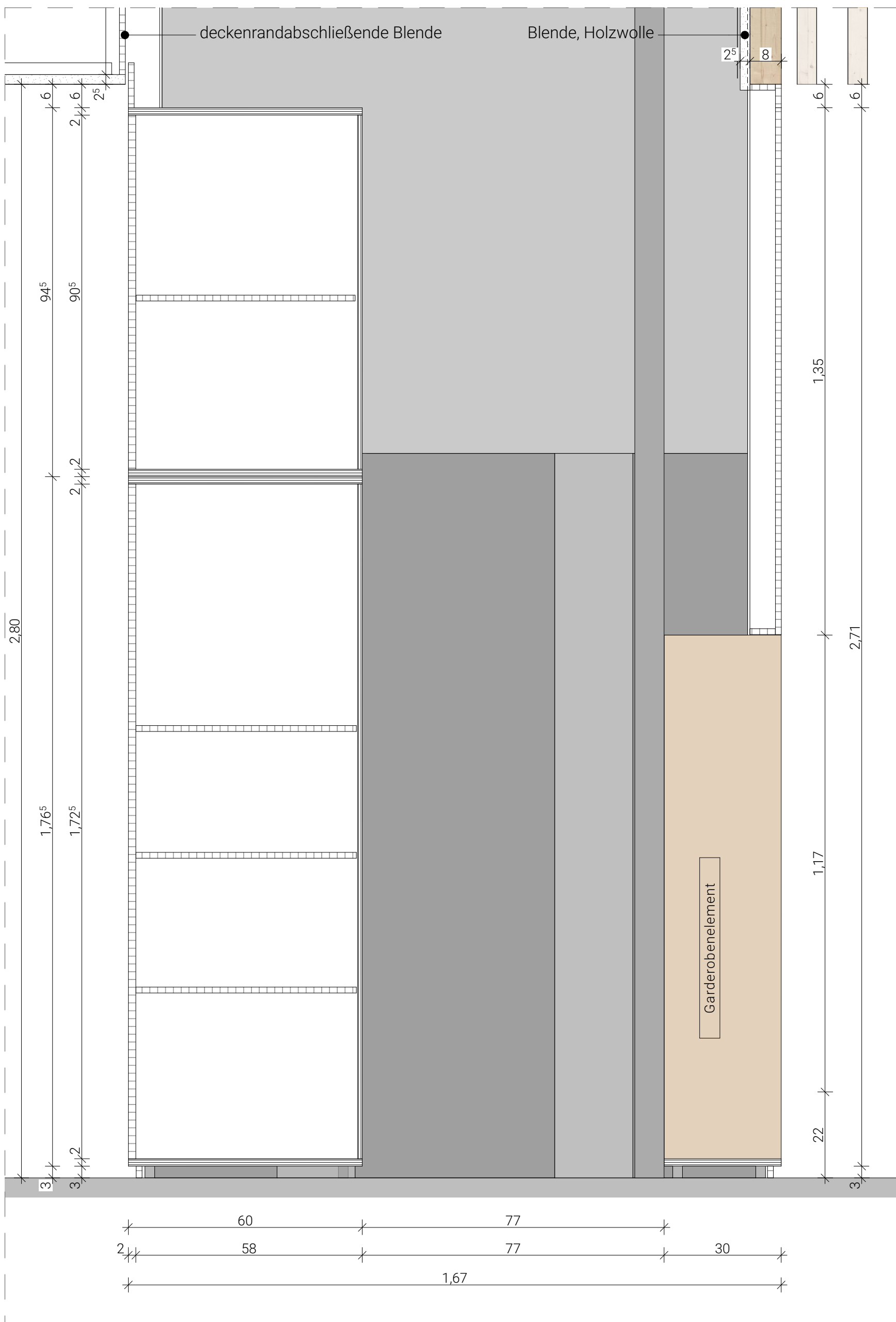
Schnitt A M 1:10
