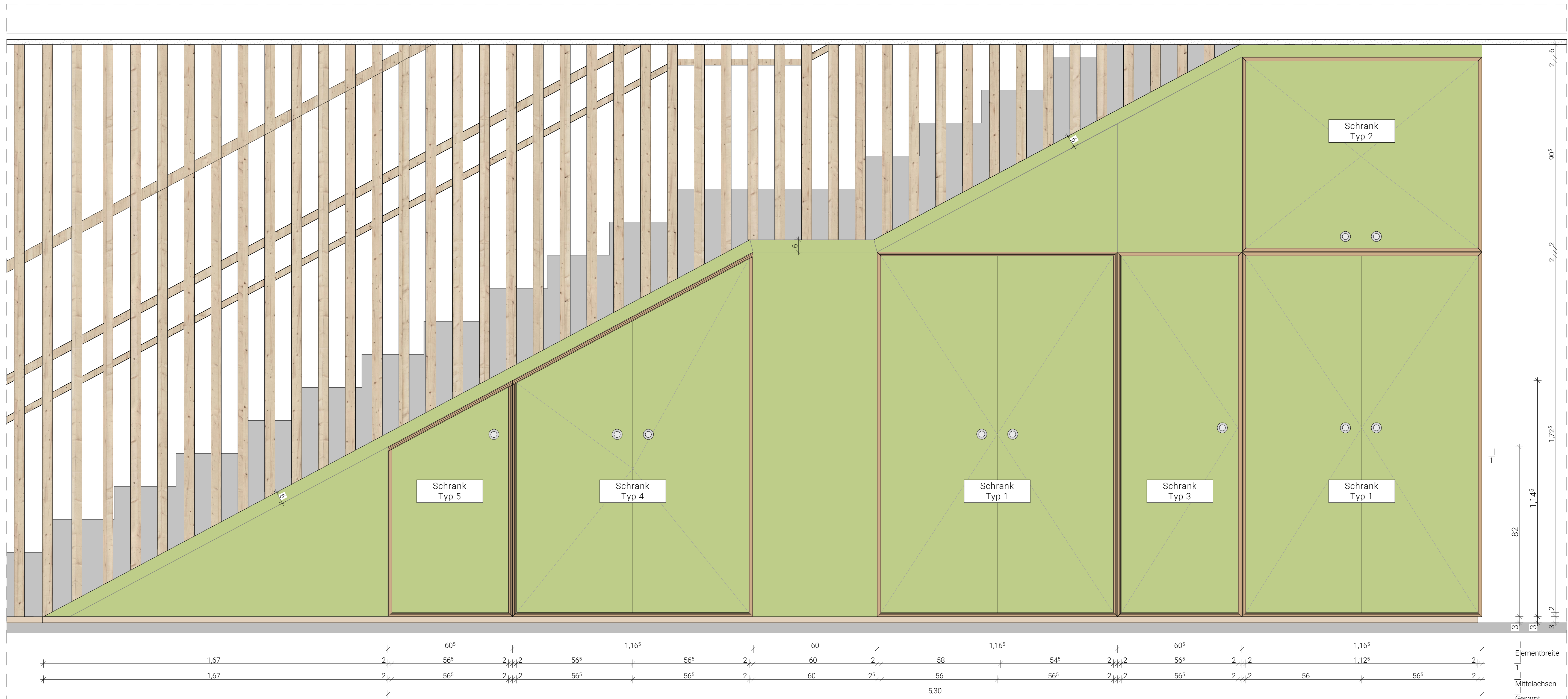
Ansicht Schrankseite M 1:10
