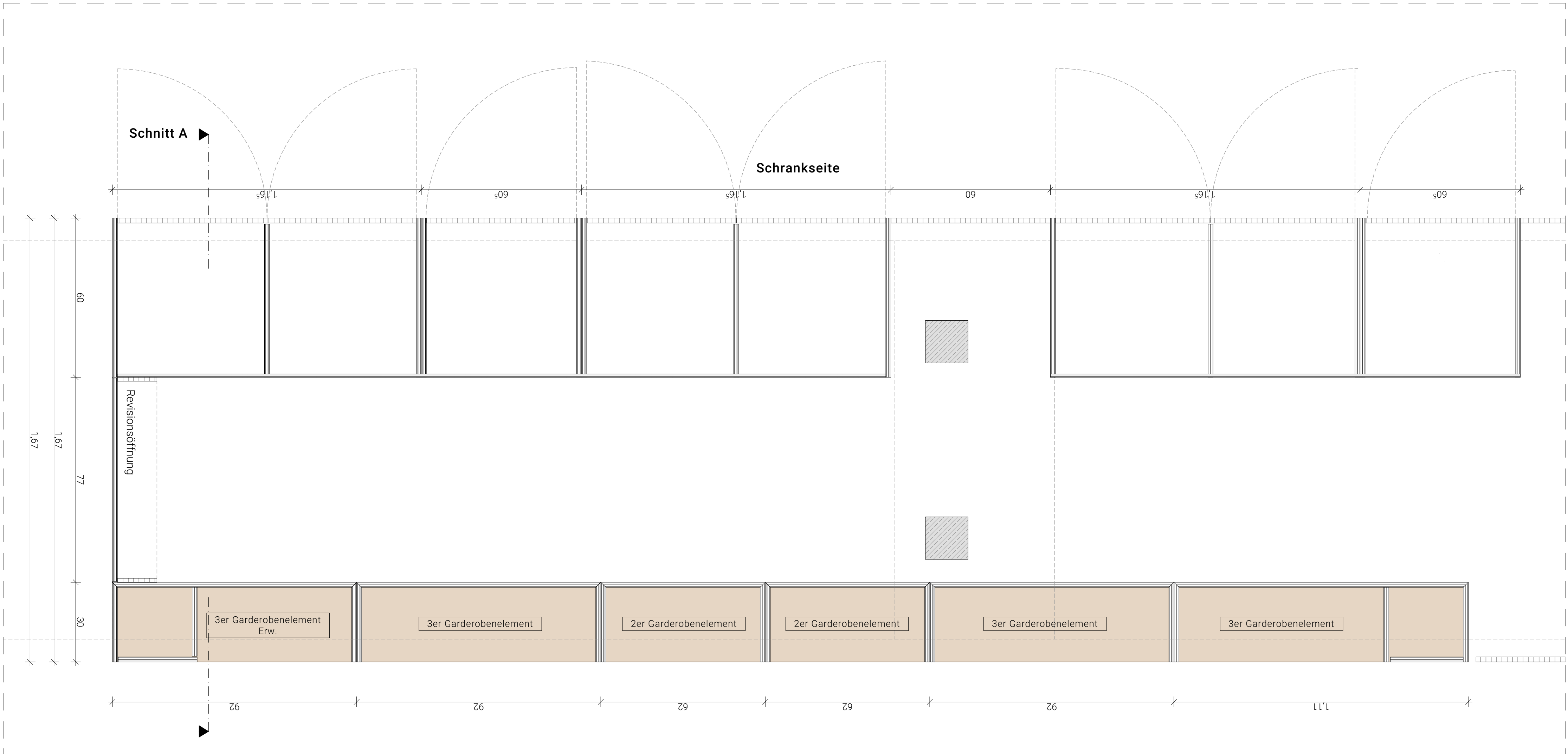
Grundriss M 1:10
