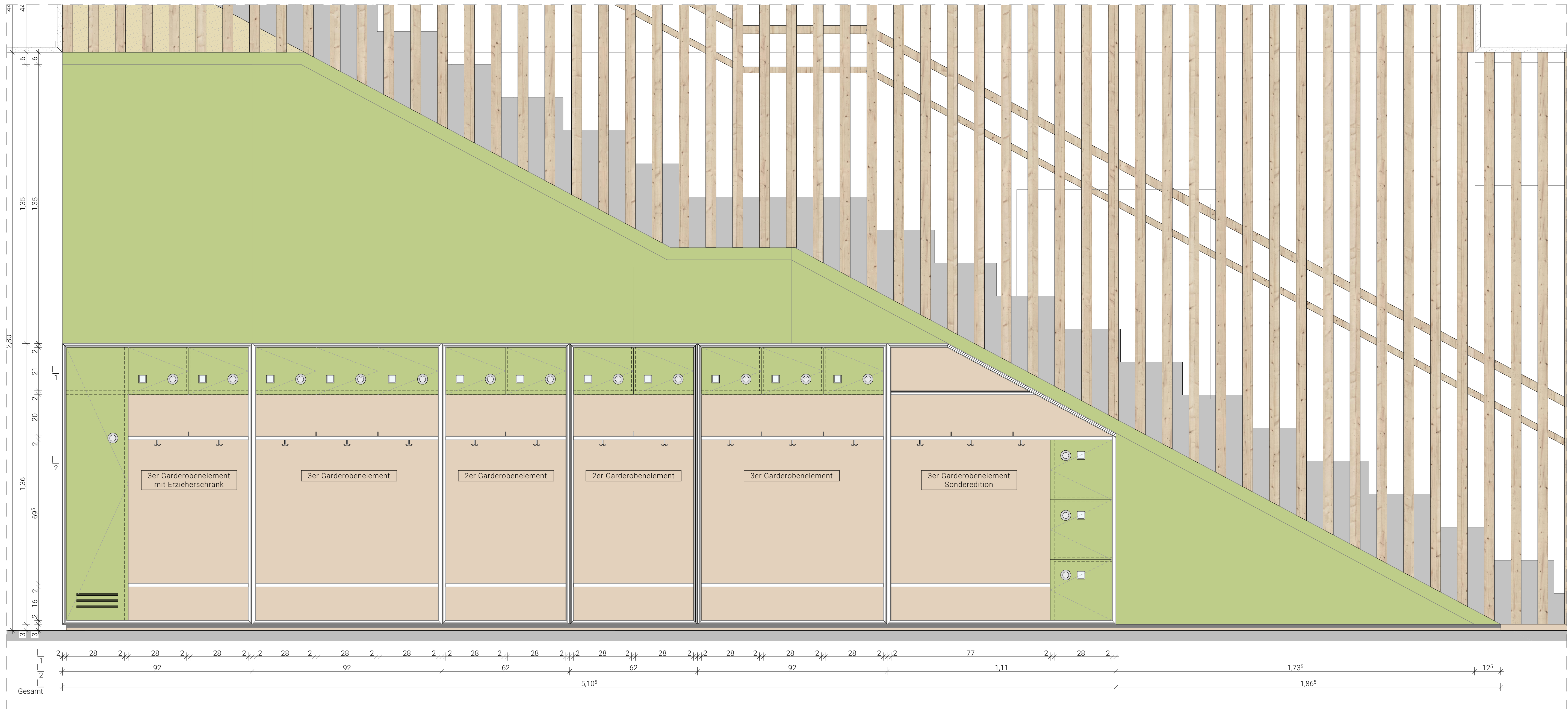
Ansicht Garderobenseite M 1:10
