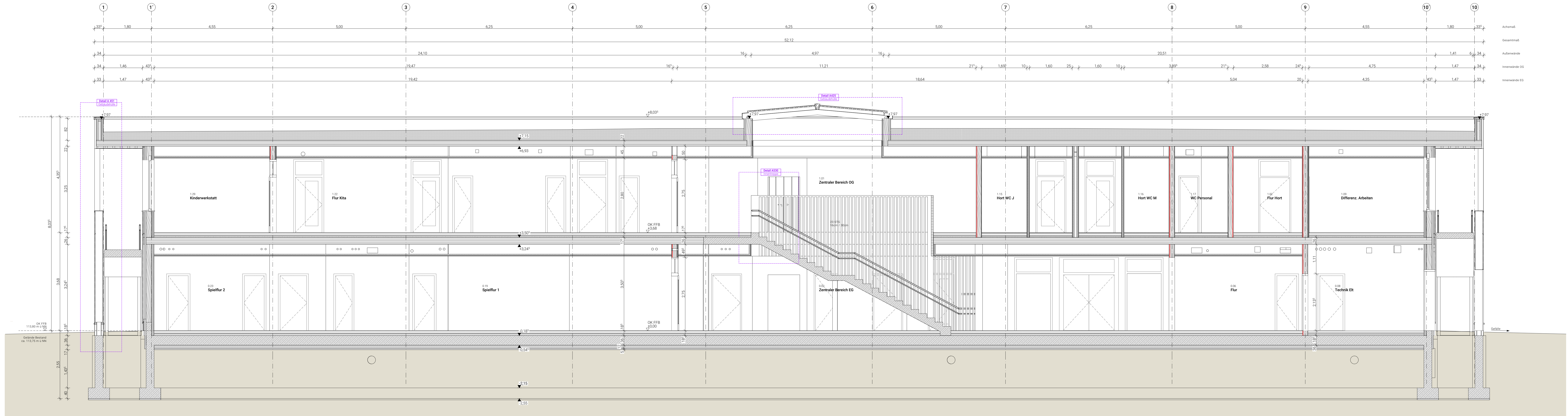
Längsschnitt A-A
