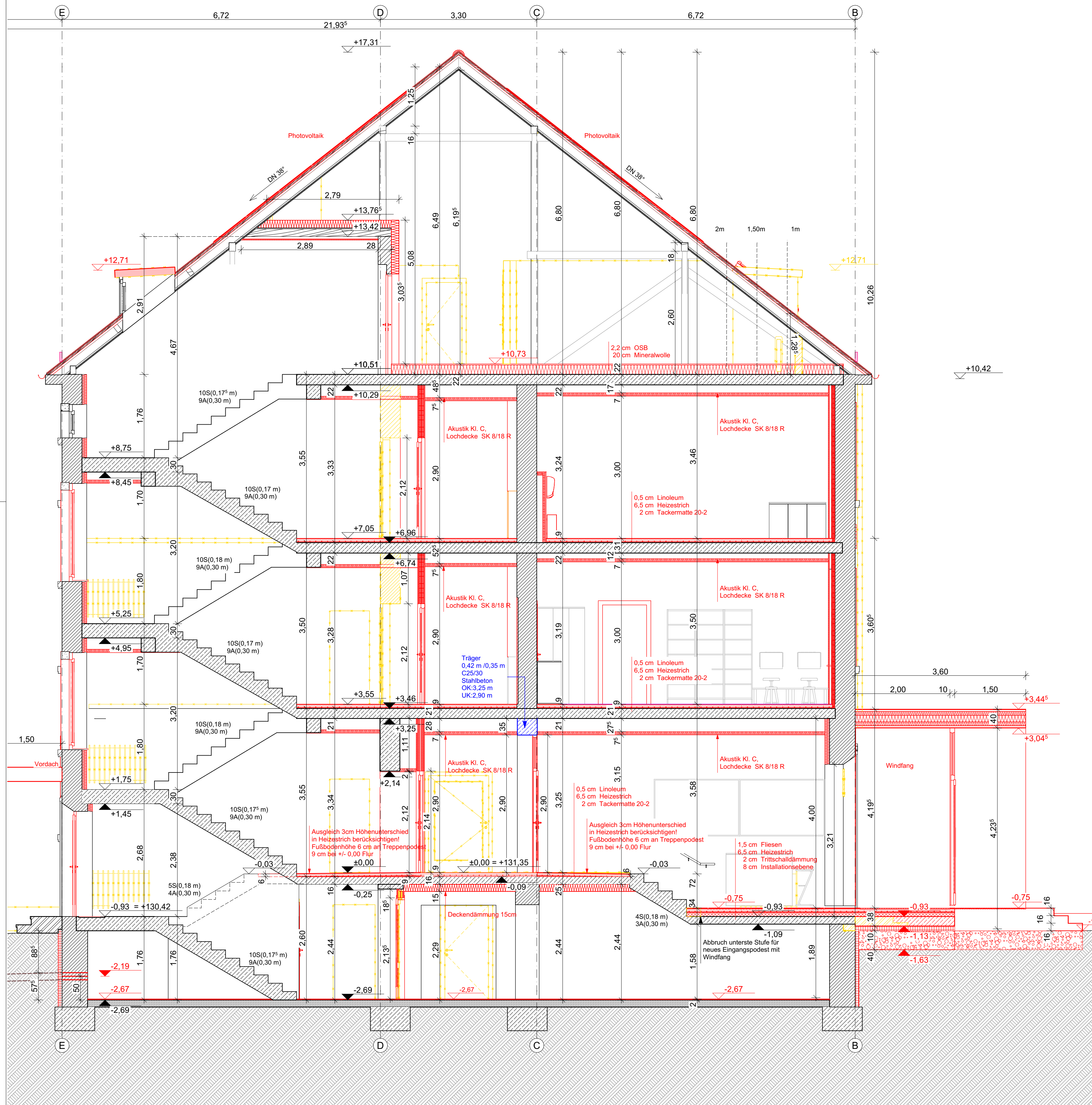
Schnitt C-C
