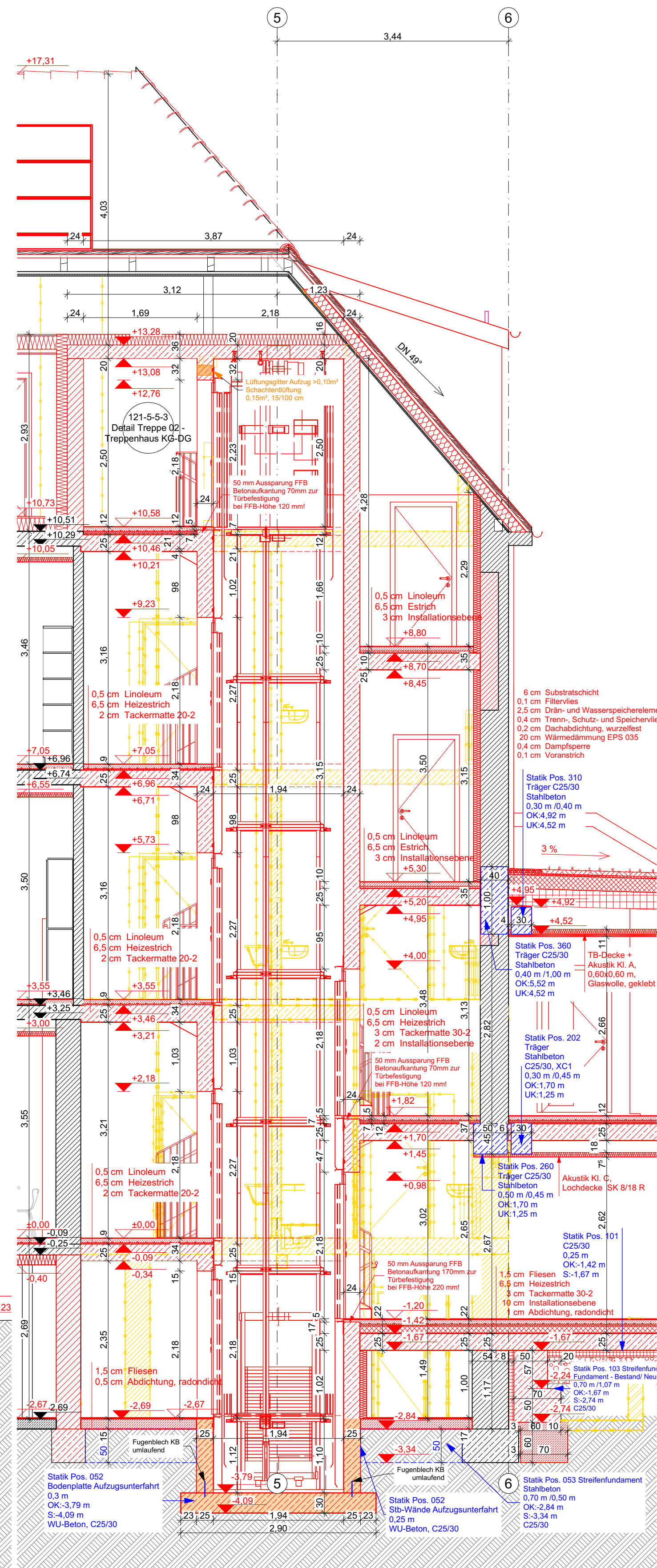
Schnitt D-D
