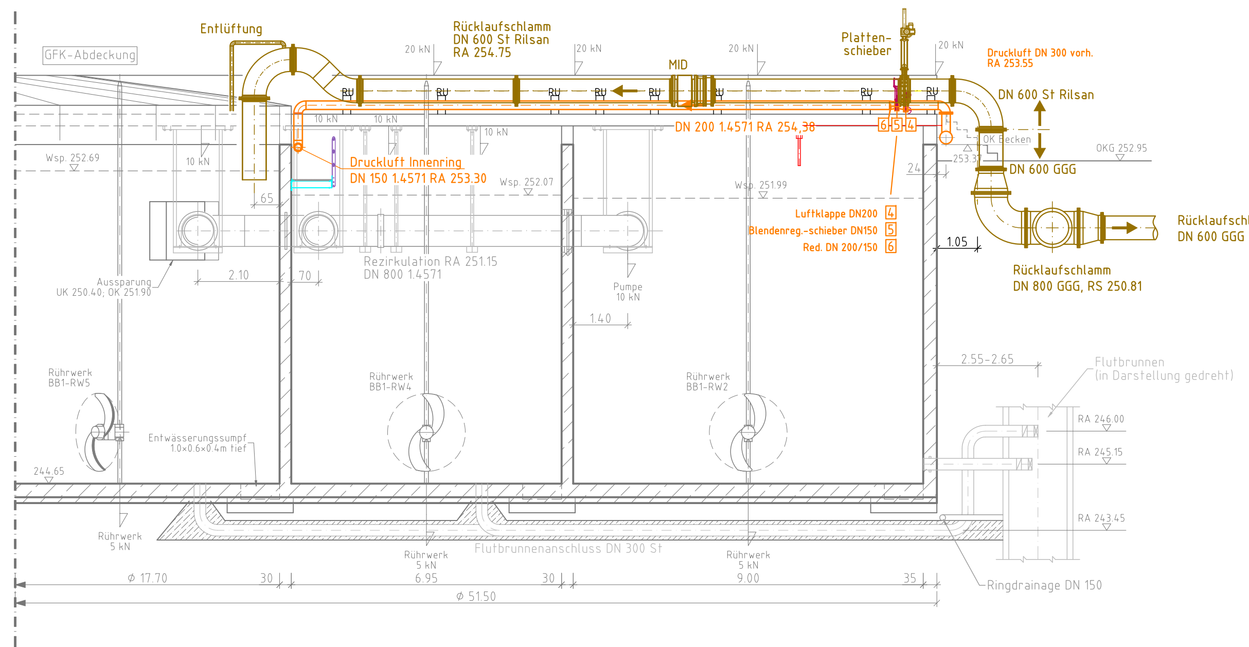
Belebungsbecken 1 Schnitt A-A - M 1:100 -Planung-
