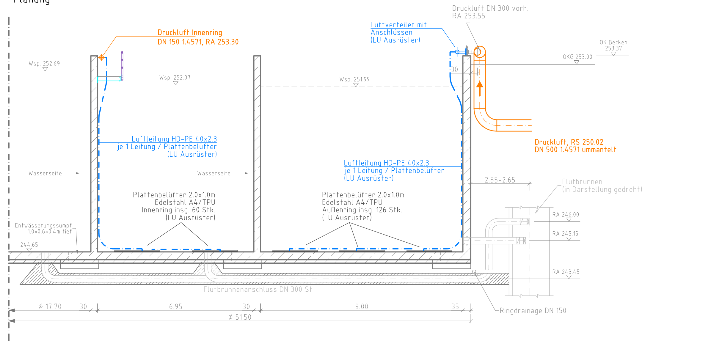
Belebungsbecken 1 Schnitt B-B - M 1:100 -Planung-
