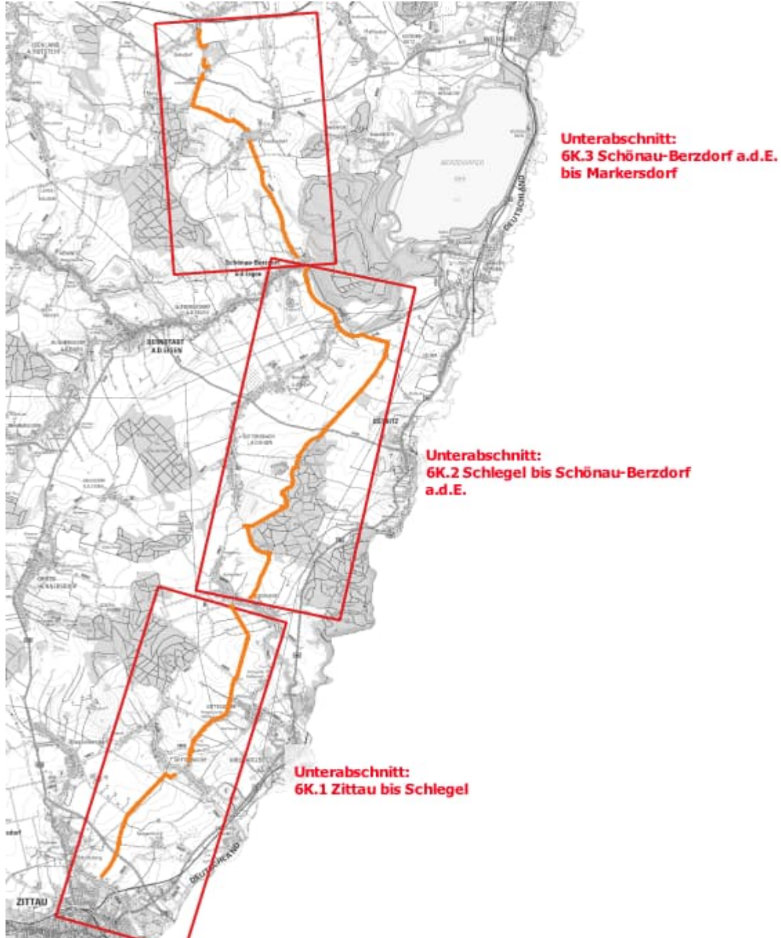
Auszug Übersichtslageplan
