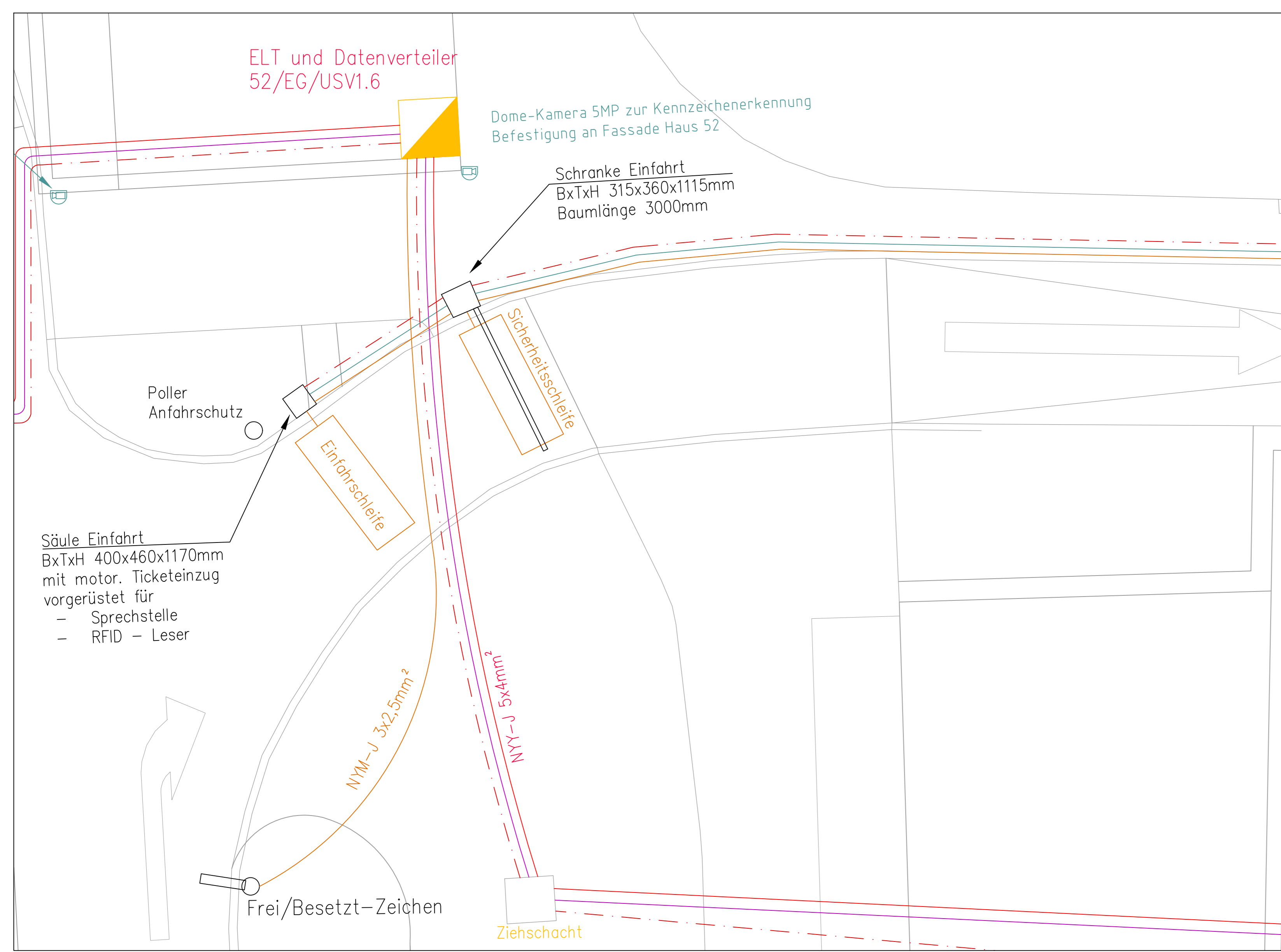
Ansicht Schrankenanlage TA00 Vorderseite/ M1:50
