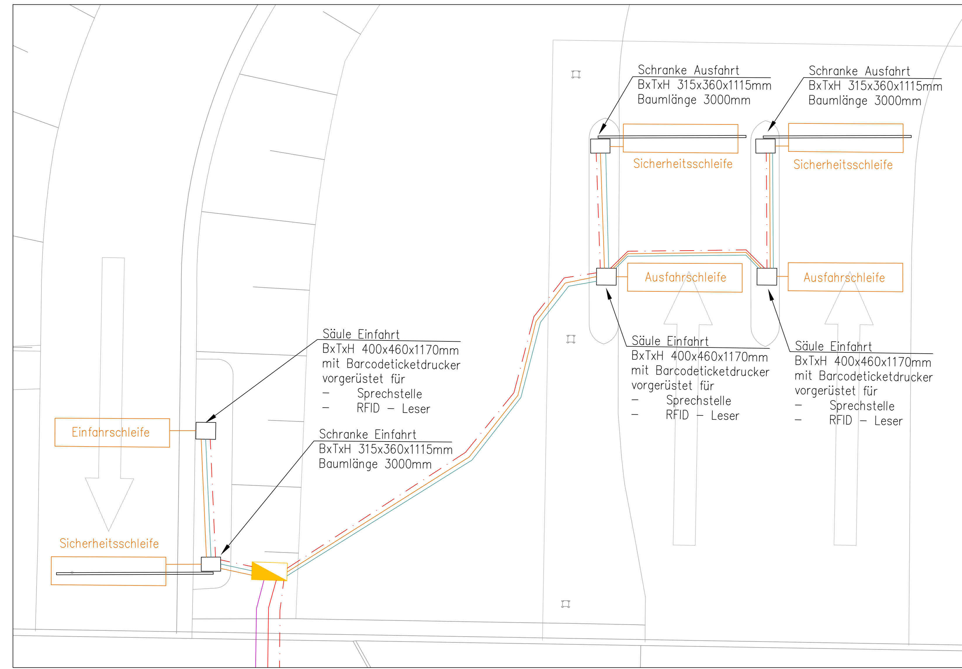
Ansicht Schrankenanlage TA00 Rückseite/ M1:50
