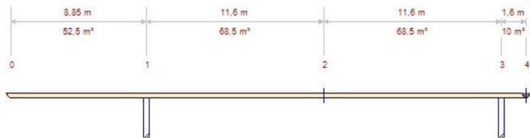
Rinnenaufteilung Westtraufe
