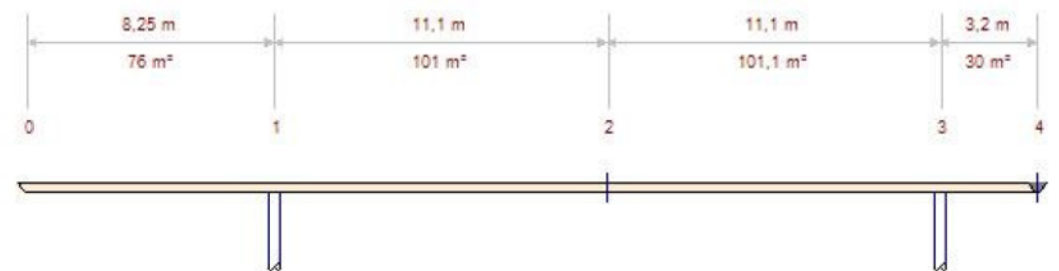
Rinnenaufteilung Osttraufe
