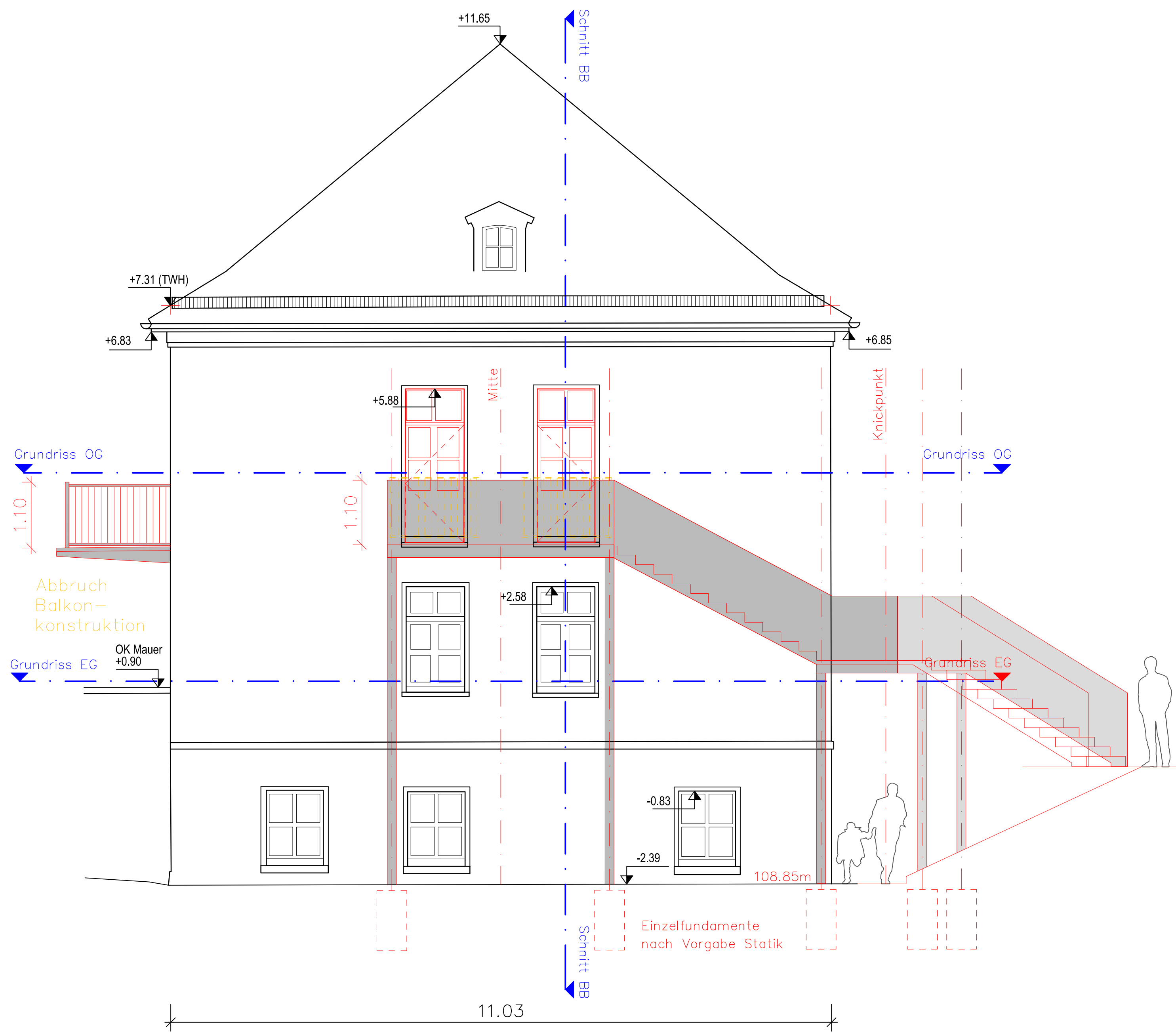
Ansicht Südost
