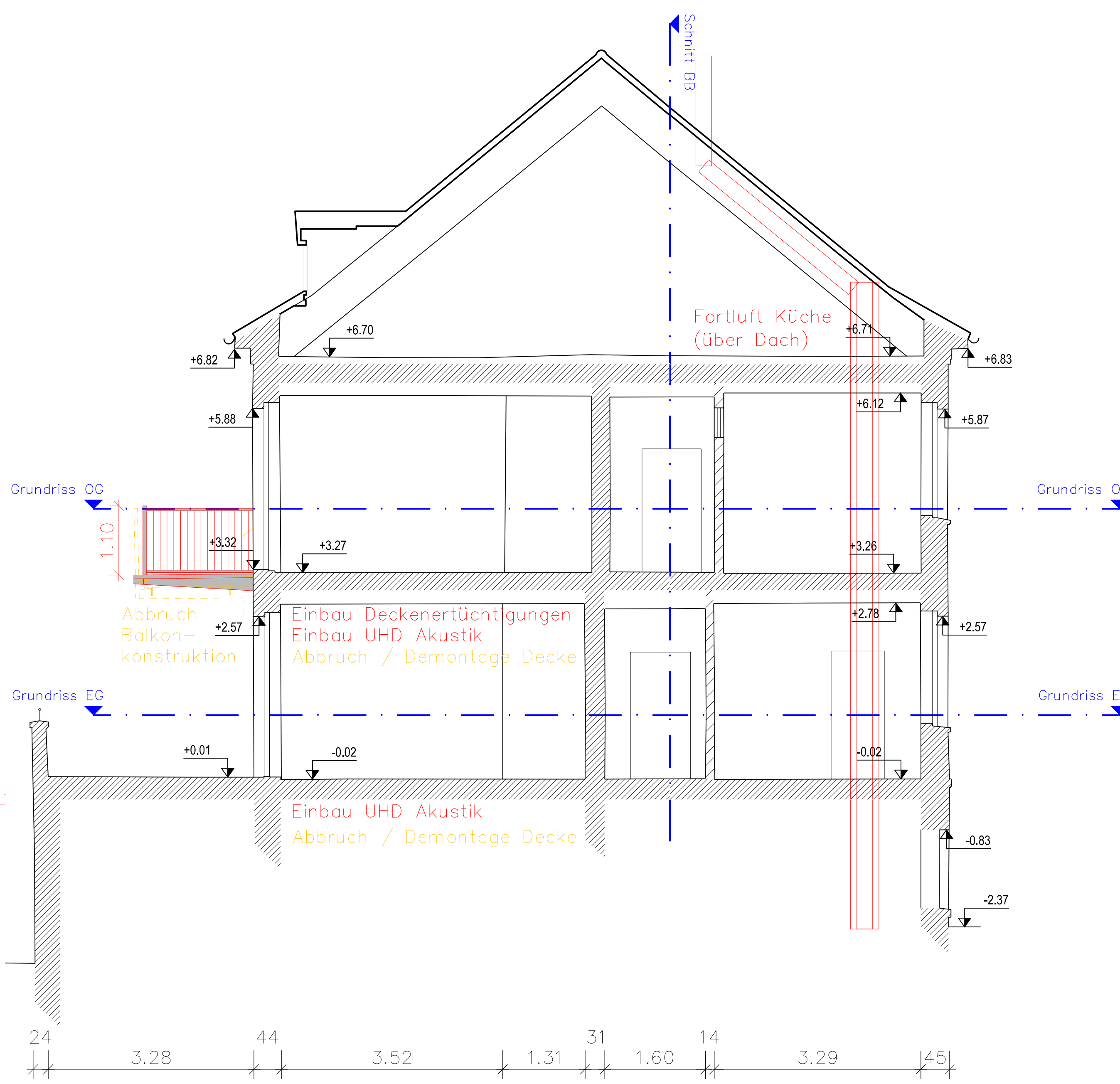
Gebäudeschnitt AA
