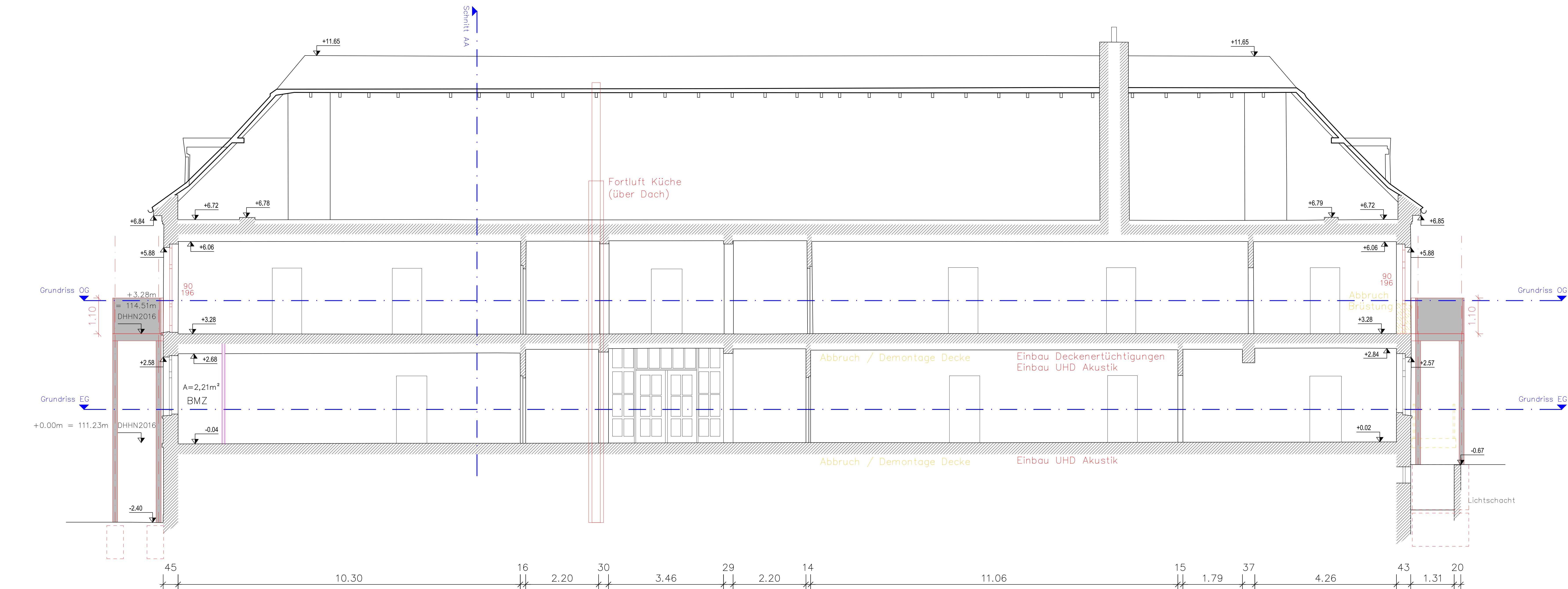
Ansicht Südost
