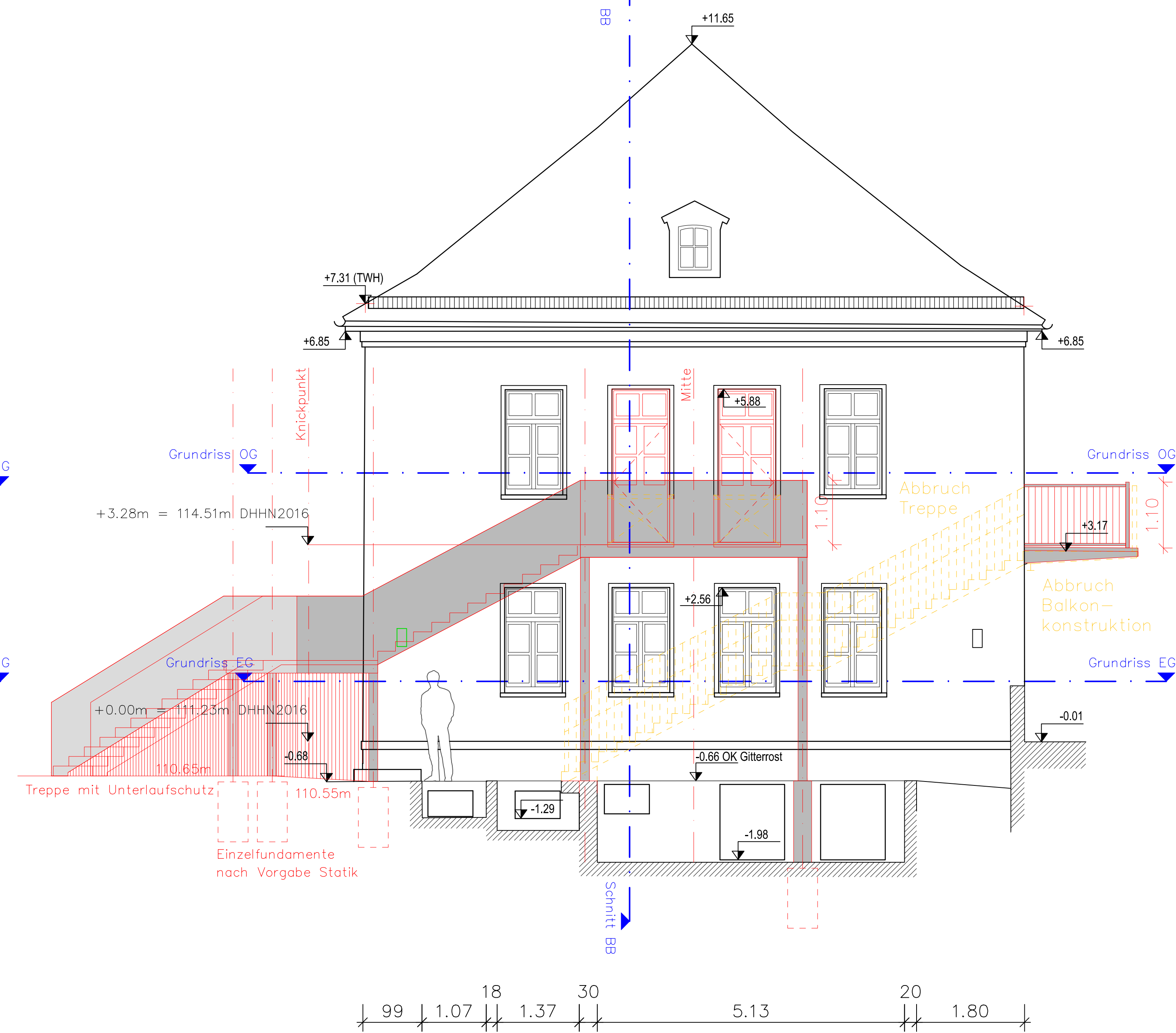
Ansicht Nordwest
