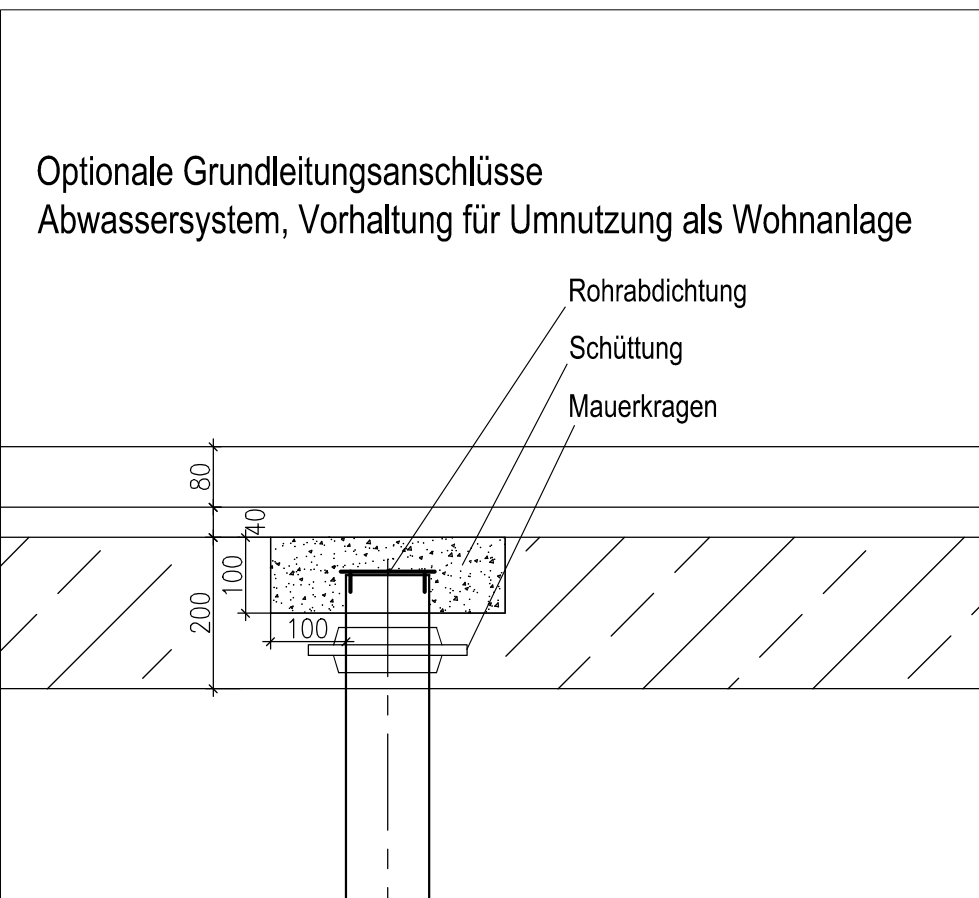
Detail Grundleitungsanschlüsse 'optionale Nutzung'
