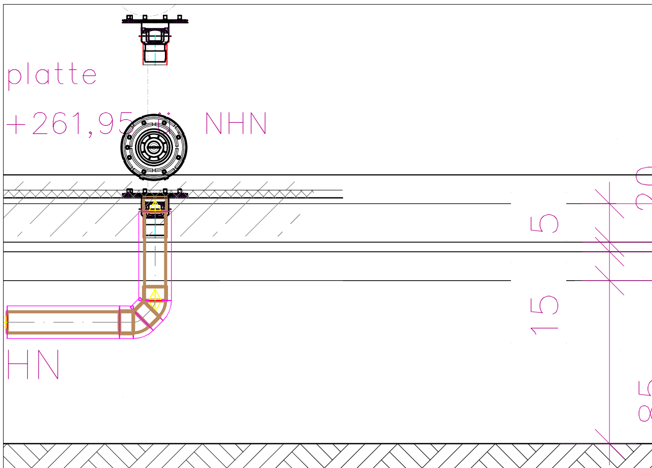
Detail Bodeneinlauf
