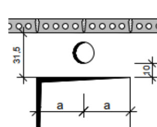
Kernbohrung über Türöffnungen
