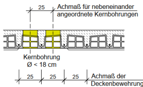
Regeldetail für Kernbohrungen
