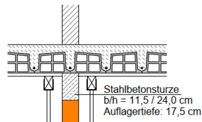
Einbau Betonstürze - Pos 4
