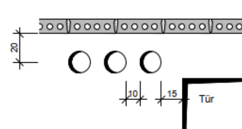
Kernbohrungen neben Türöffnungen
