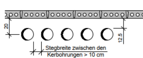
Kernbohrungen ohne Sturz
