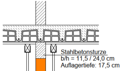
Einbau Betonstütze -
