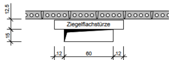
Wandöffnungen mit Sturz
