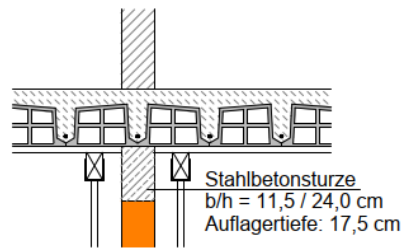
Einbau Betonstürze - Pos 4
