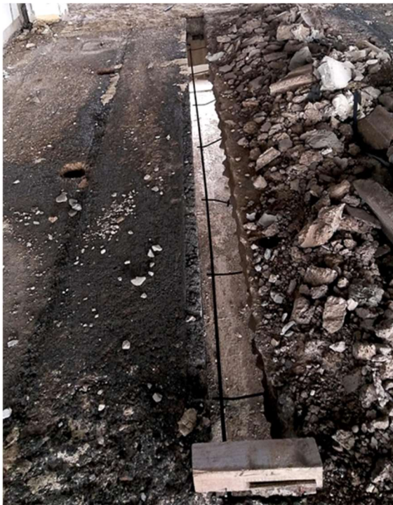
Abbildung 8: Pos. 3..10 – Sicherung von Fehlstellen, Durchbrüchen in Stahlbeton
